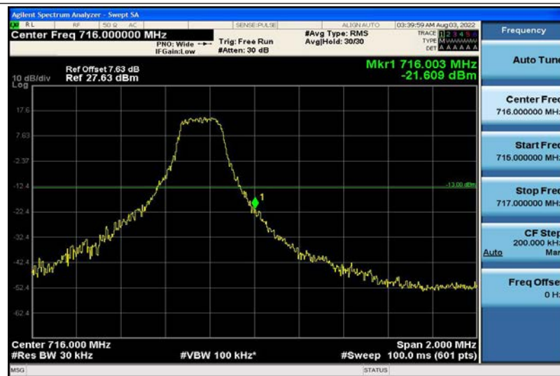
Band12-3MHz-QPSK-23165-1RB#14
