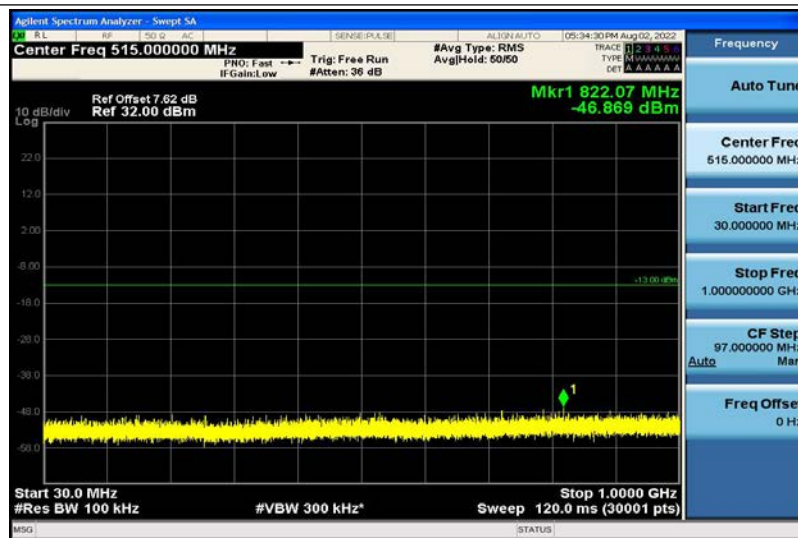
Band2-20MHz-QPSK-18700-1RB#0-30~1000MHz
