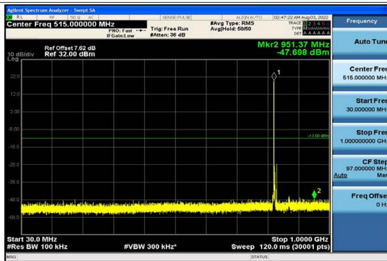
Band5-5MHz-QPSK-20425-1RB#0-30~1000MHz
