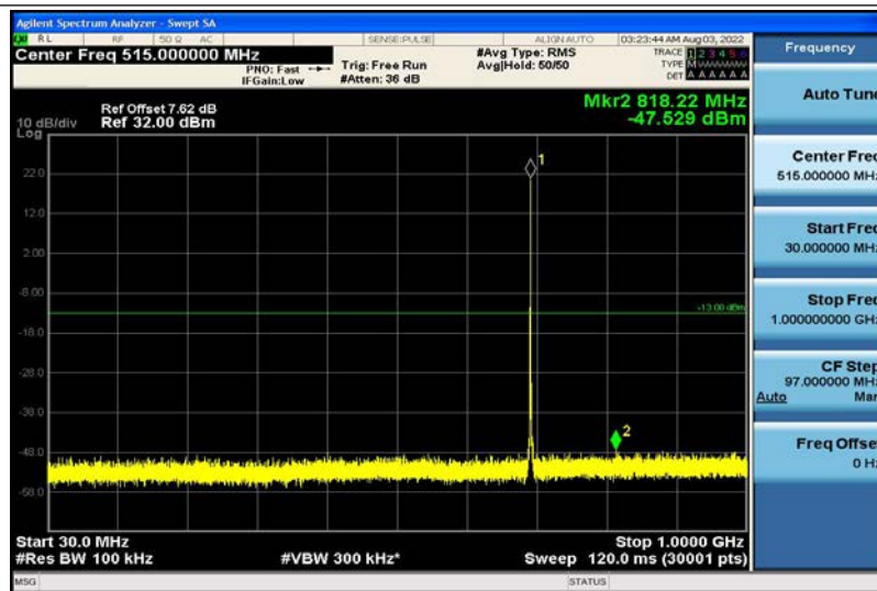
Band12-1.4MHz-QPSK-23017-1RB#0-30~1000MHz
