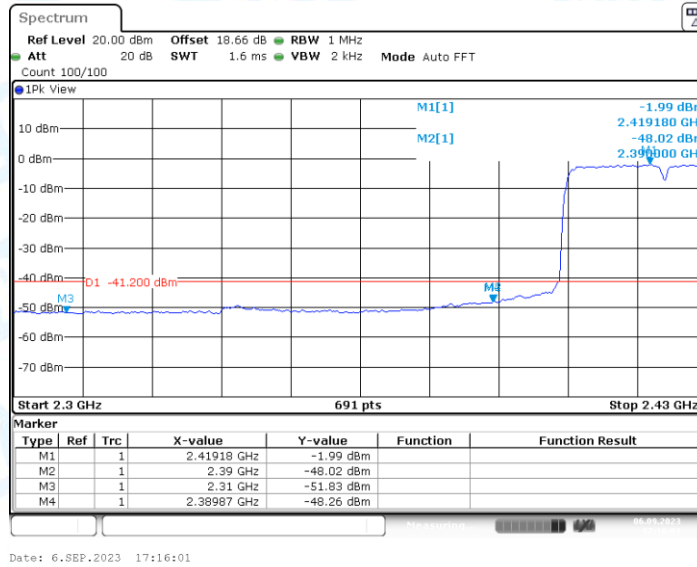
11N40MIMO_Ant1_Low_2422_Peak
