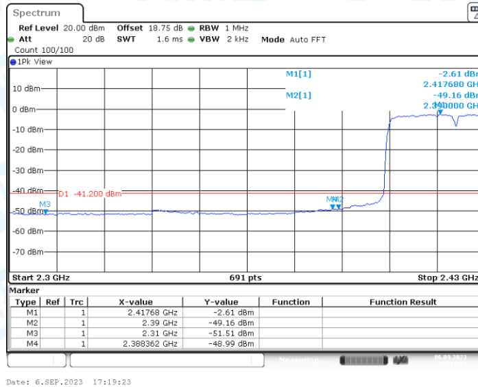
11N40MIMO_Ant2_Low_2422_Peak
