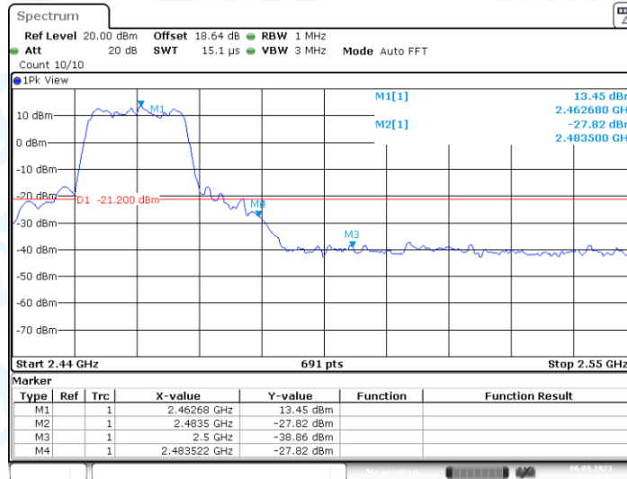
11N20MIMO_Ant2_High_2462_AV
