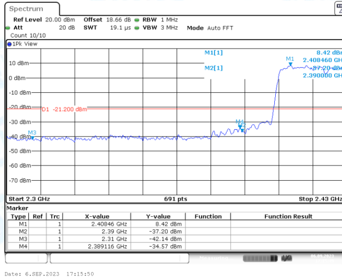
11N40MIMO_Ant2_Low_2422_AV
