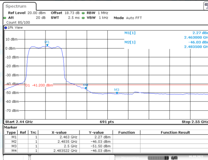
11N20MIMO_Ant2_High_2462_AV
