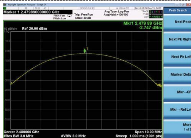
GFSK(CH78)
