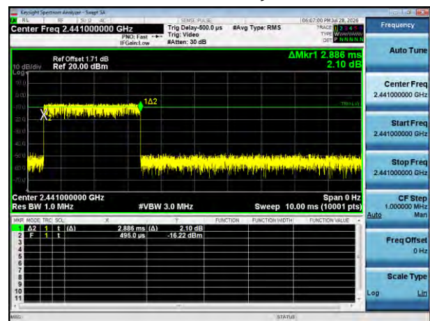
Burst2DH5)
