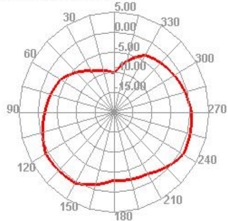
2470.000MHz H
