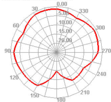
2450.000MHz E2
