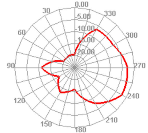
5500.000MHz E2
