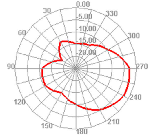
5500.000MHz H
