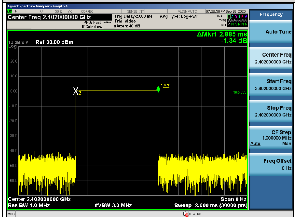
Test_Graph_2.4G_HOP_ANT1_NA_GFSK_2402_Time per Burst
