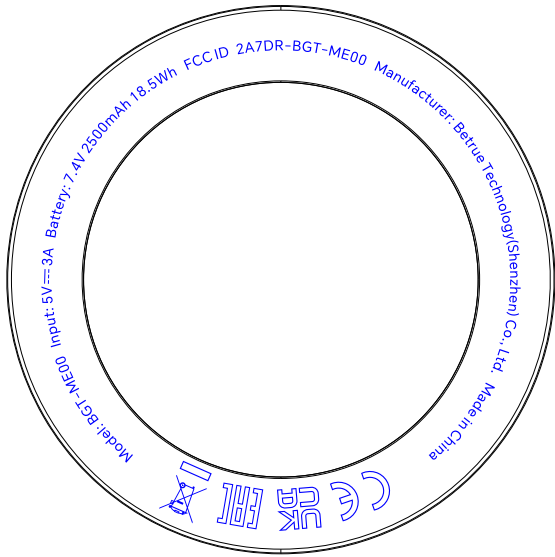
被动盘底部丝印方向在整个机器上位置示意 铭牌信息丝印光油参考样品的效果
