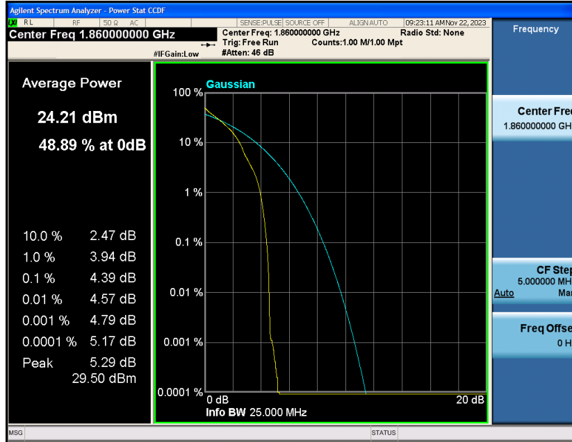
Band2-20MHz-QPSK-18700-100RB#0
