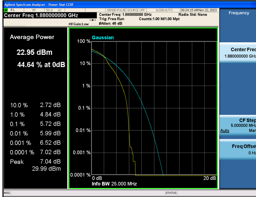
Band2-20MHz-16QAM-18900-100RB#0
