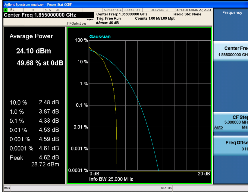
Band2-10MHz-QPSK-18650-50RB#0
