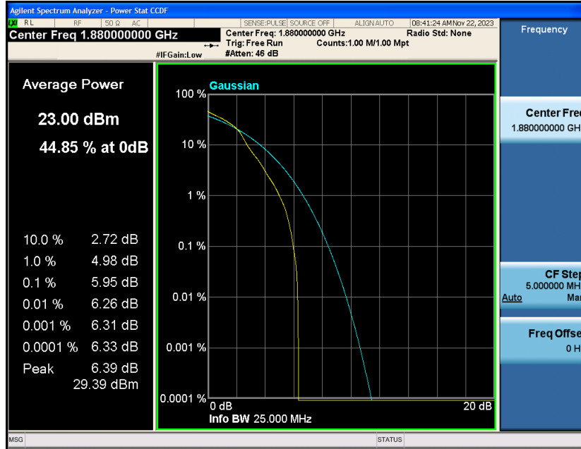
Band2-10MHz-16QAM-18900-50RB#0
