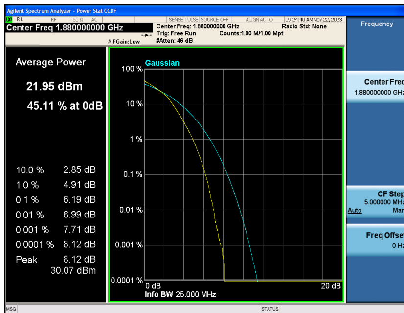
Band2-20MHz-16QAM-19100-1RB#0
