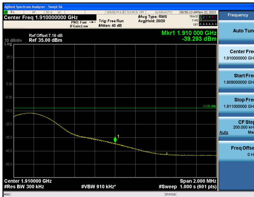
Band2-15MHz-16QAM-19125-1RB#74
