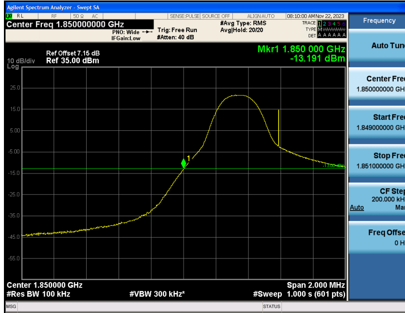
Band2-5MHz-QPSK-18625-1RB#24
