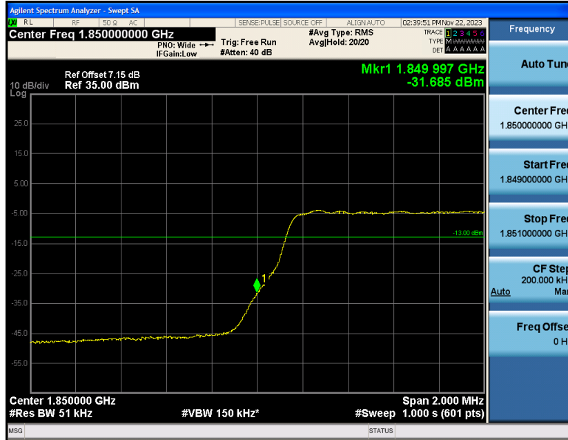
Band2-3MHz-QPSK-19185-1RB#0
