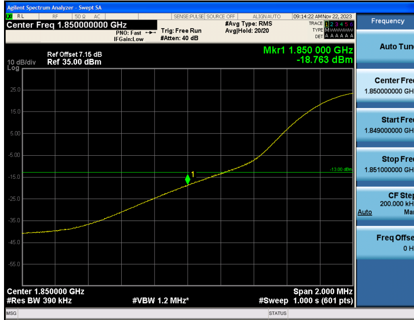
Band2-20MHz-QPSK-18700-1RB#99
