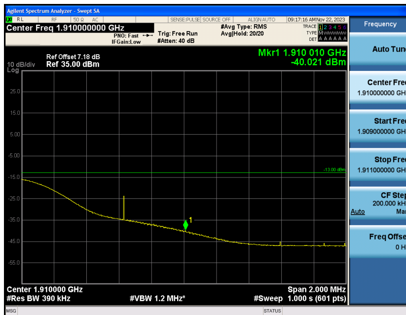
Band2-20MHz-QPSK-19100-1RB#99
