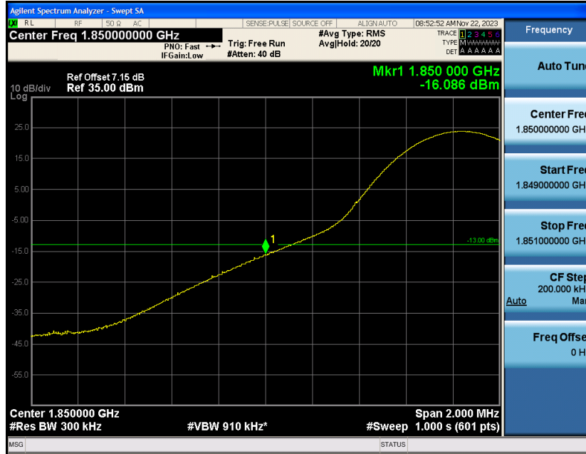
Band2-15MHz-QPSK-18675-1RB#74
