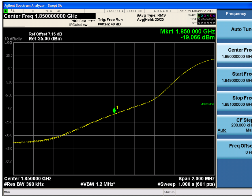
Band2-20MHz-16QAM-18700-1RB#99
