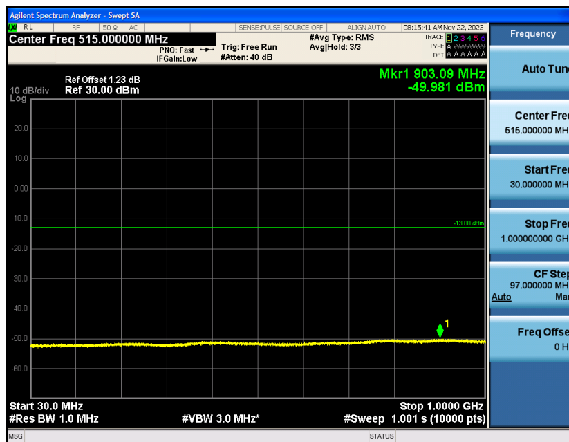
Band2-5MHz-QPSK-18625-1RB#0-Range2:1000~20000MHz
