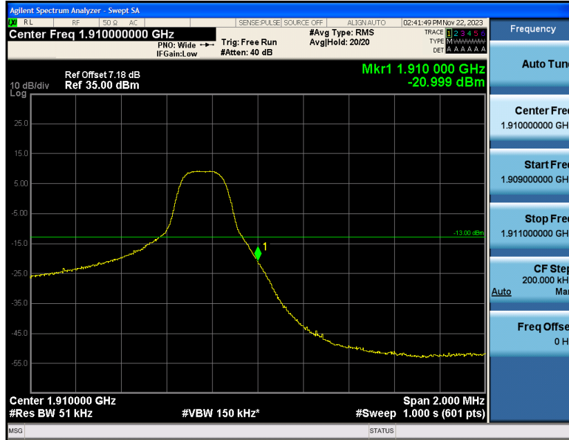
Band2-3MHz-QPSK-19185-15RB#0
