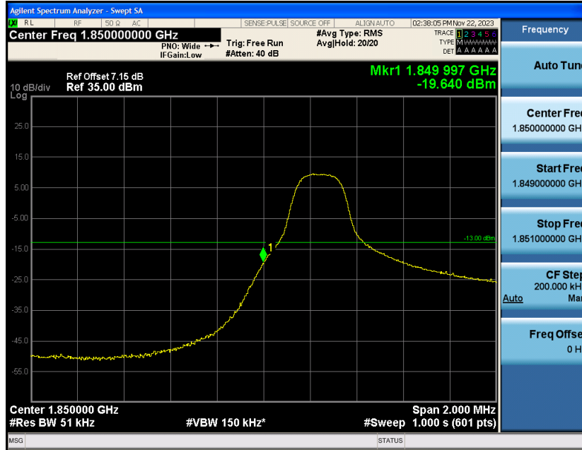
Band2-3MHz-QPSK-18615-1RB#14
