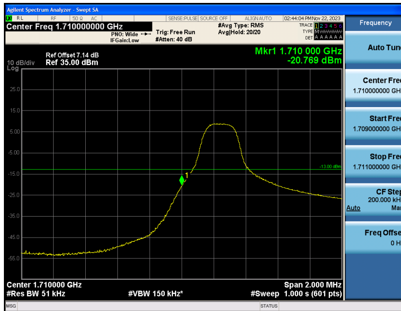
Band4-3MHz-QPSK-19965-1RB#14
