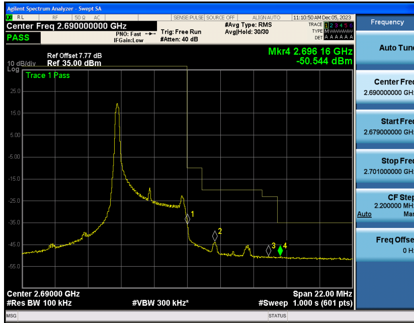
Band41-5MHz-16QAM-41565-1RB#24
