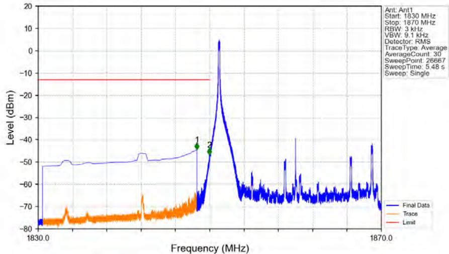
Band2_20MHz_QPSK_LCH_1860MHz_RB_1_0_NTNV
