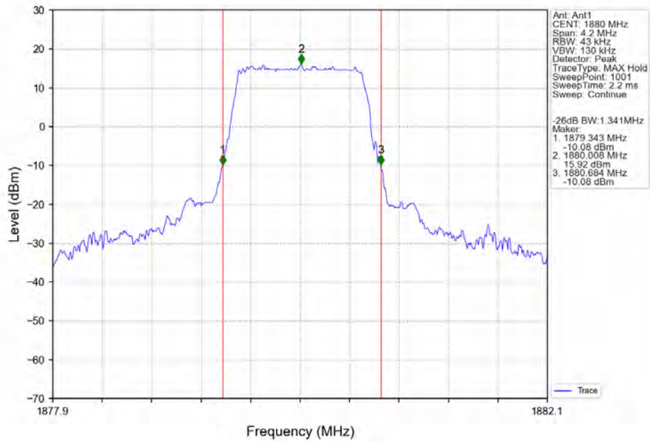
Band2 1.4MHz QPSK MCH 1880MHz RB 6 0 NTN
