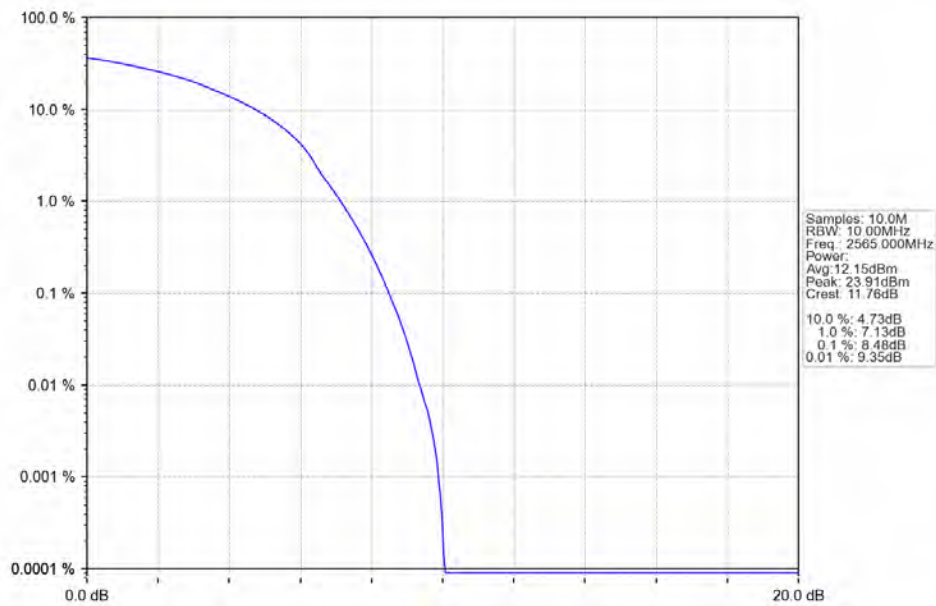
Band41_20MHz_16QAM_LCH_2565MHz_RB_100_0_NTNV
