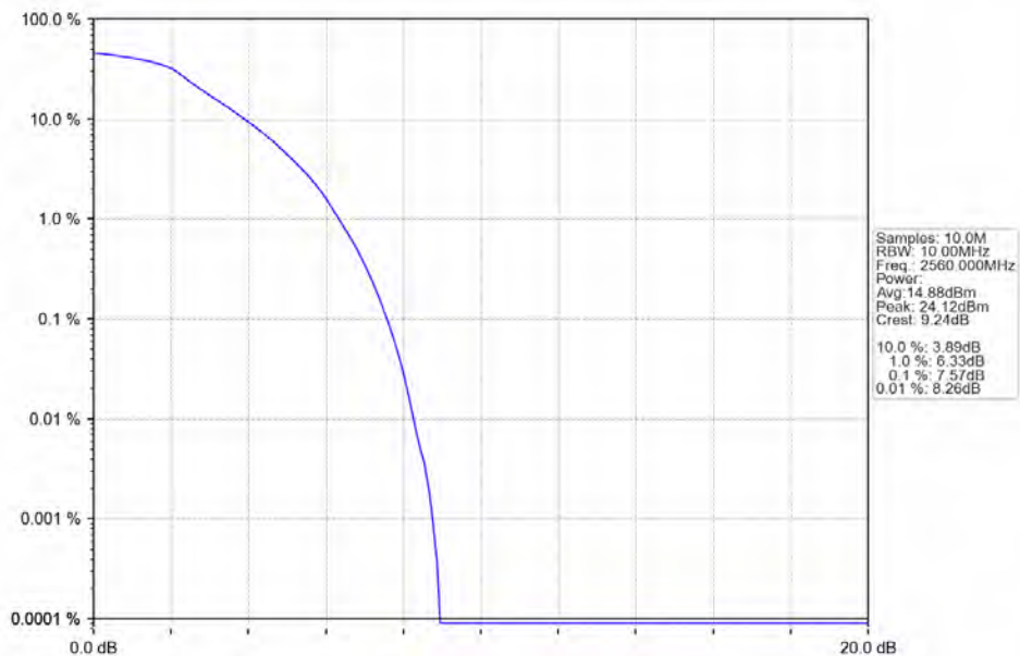
Band41_10MHz_QPSK_LCH_2560MHz_RB_50_0_NTNV
