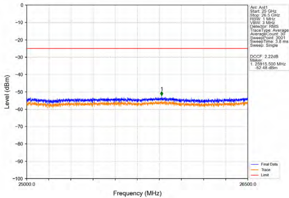
Band41_10MHz_16QAM_LCH_2560MHz_RB_50_0_NTNV
