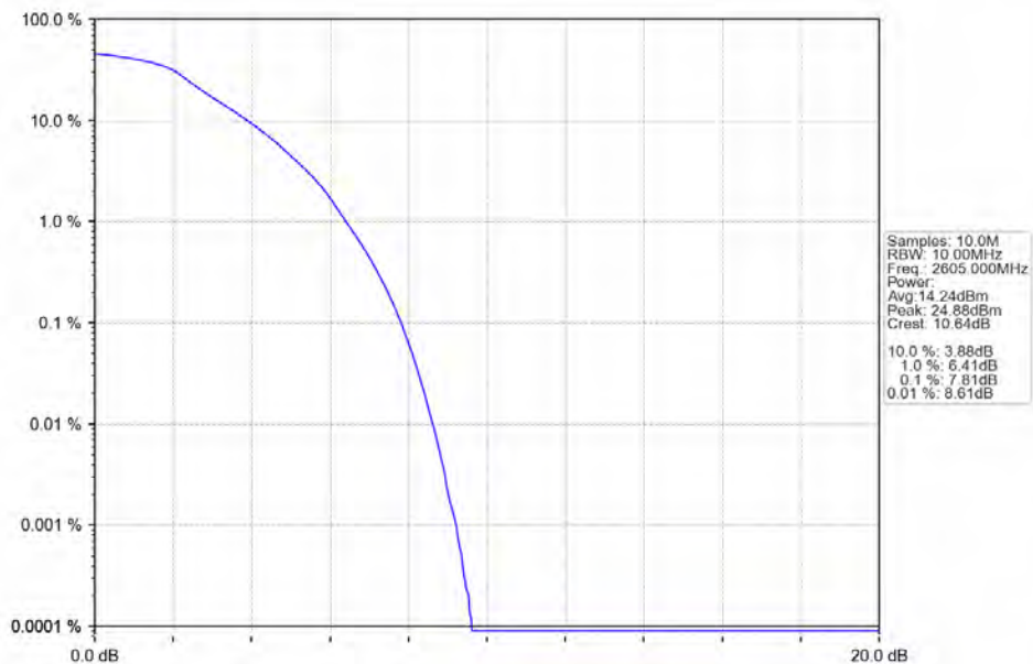
Band41_10MHz_QPSK_MCH_2605MHz_RB_50_0_NTNV
