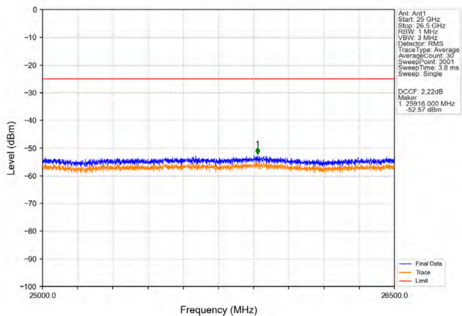
Band41_5MHz_QPSK_LCH_2557.5MHz_RB_1_0_NTNV
