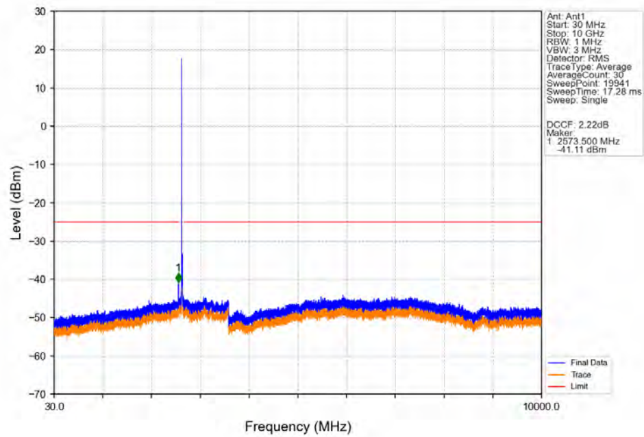
Band41_20MHz_QPSK_HCH_2645MHz_RB_1_0_NTNV
