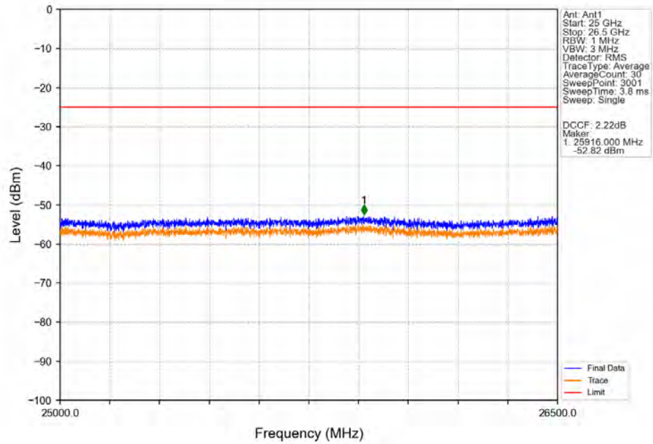
Band41_15MHz_QPSK_HCH_2647.5MHz_RB_1_74_NTNV
