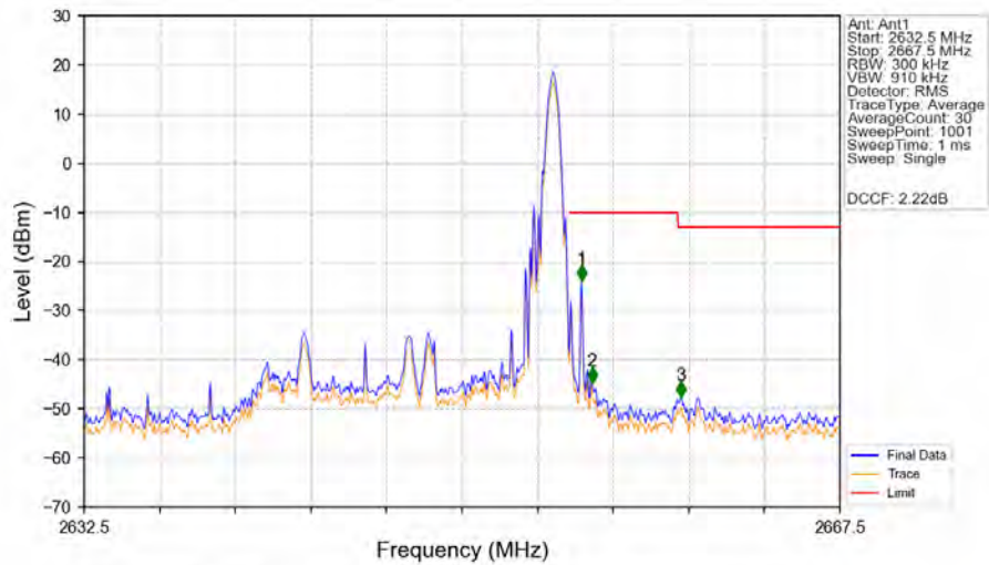
Band41_15MHz_QPSK_HCH_2647.5MHz_RB_1_74_NTNV
