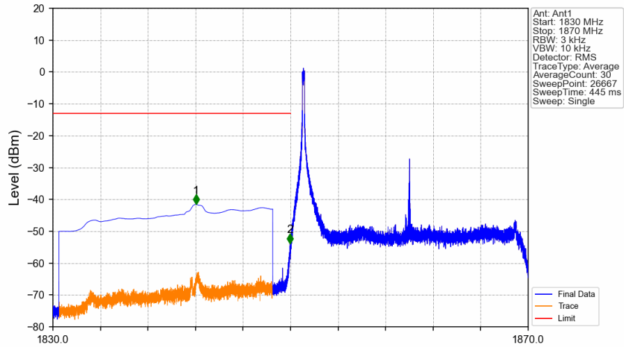
Band2_20MHz_16QAM_LCH_1860MHz_RB_1_0_NTNV
