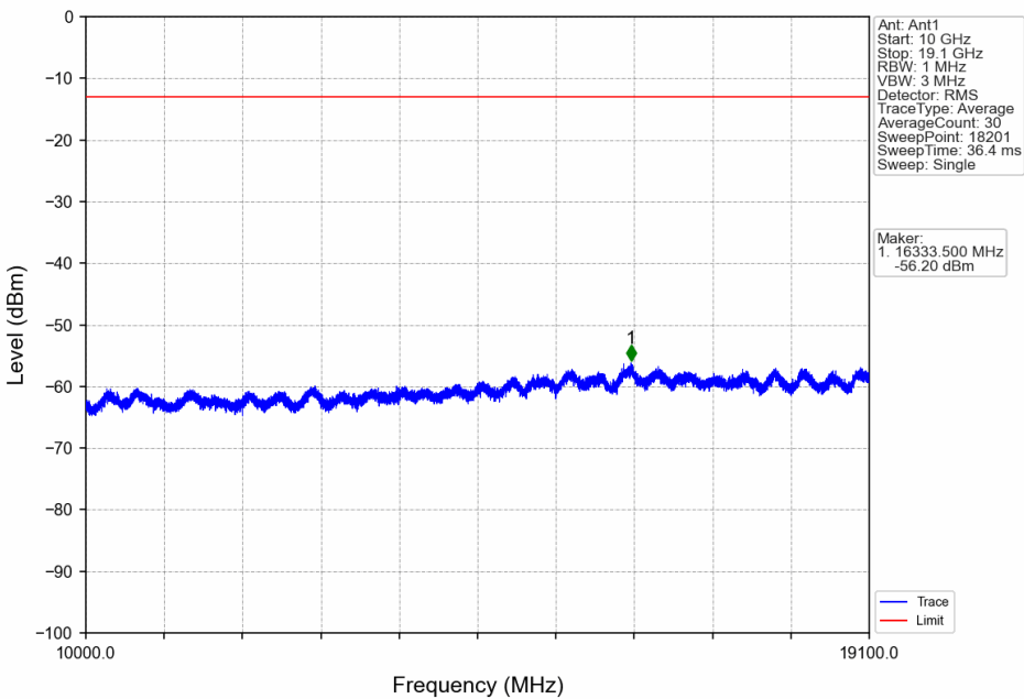
Band2_20MHz_16QAM_LCH_1860MHz_RB_100_0_NTNV
