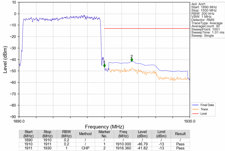
Band2_20MHz_QPSK_HCH_1900MHz_RB_100_0_NTNV
