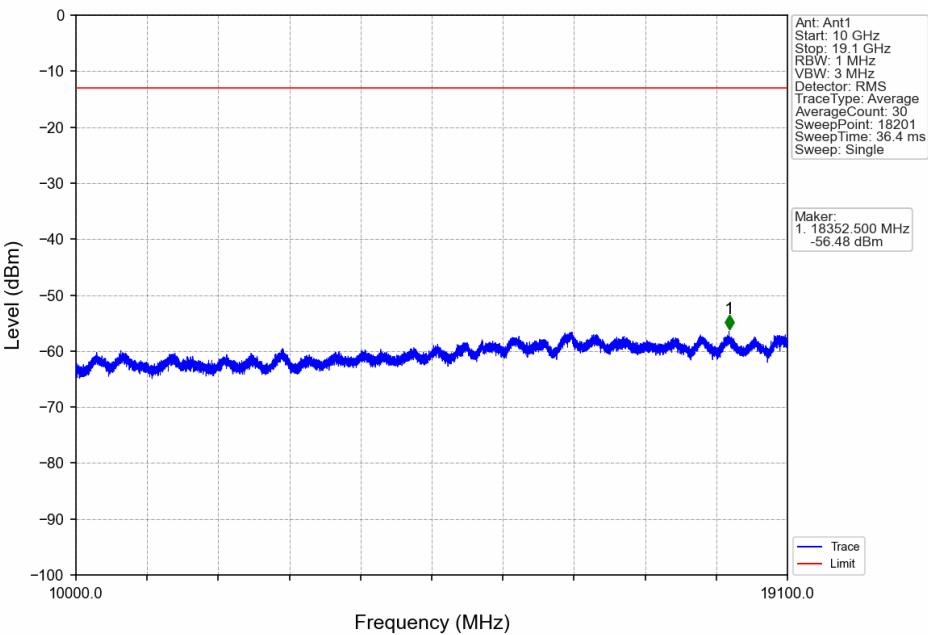
Band2_10MHz_QPSK_LCH_1855MHz_RB_50_0_NTNV
