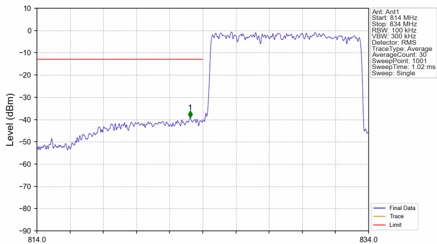
Band5_10MHz_QPSK_LCH_829MHz_RB_50_0_NTNV
