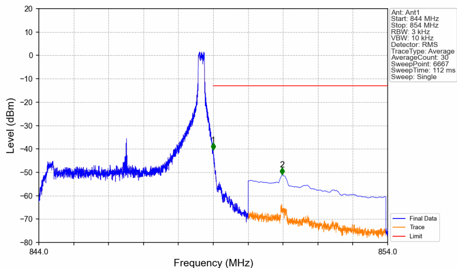
Band5_5MHz_QPSK_HCH_846.5MHz_RB_1_24_NTNV
