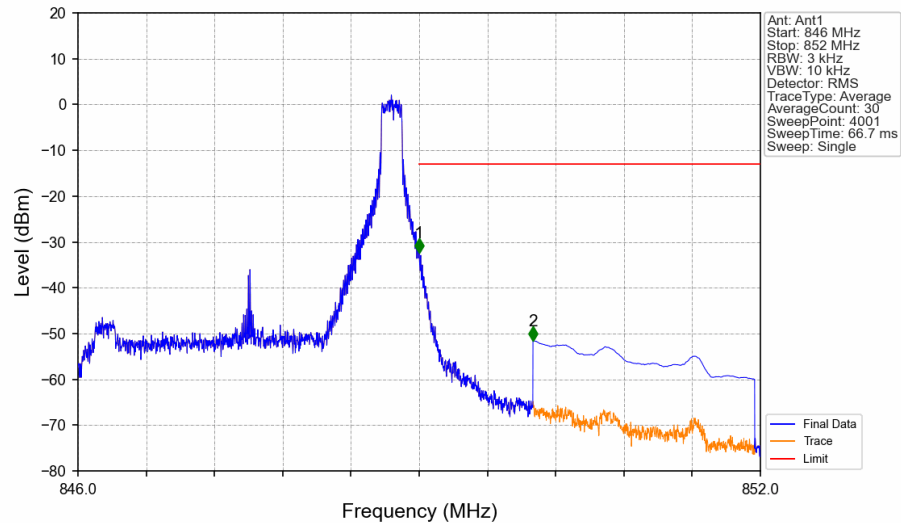
Band5_3MHz_QPSK_HCH_847.5MHz_RB_1_14_NTNV
