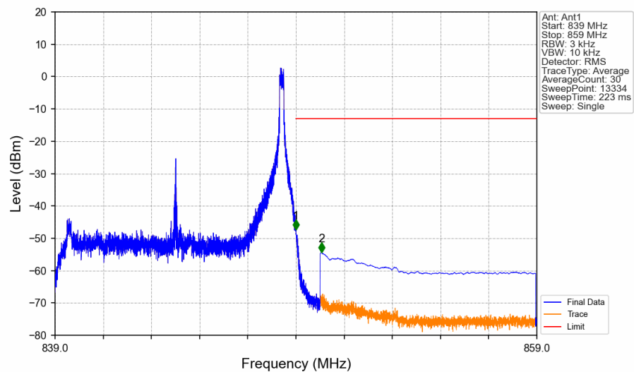
Band5_10MHz_QPSK_HCH_844MHz_RB_1_49_NTNV
