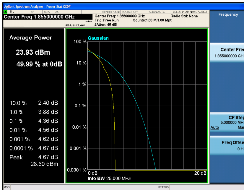
Band2-10MHz-QPSK-18650-50RB#0
