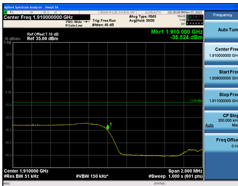
Band2-3MHz-QPSK-19185-1RB#14
