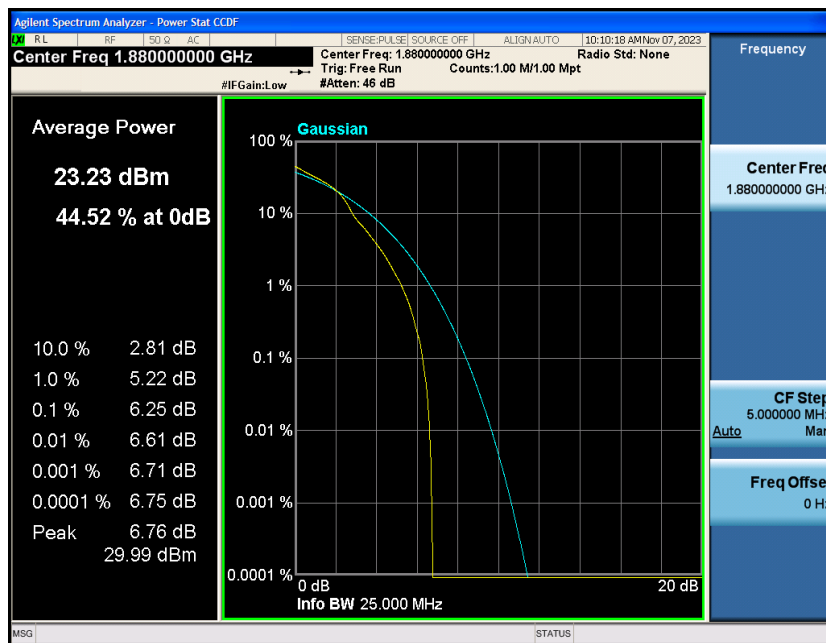
Band2-20MHz-16QAM-18900-100RB#0
