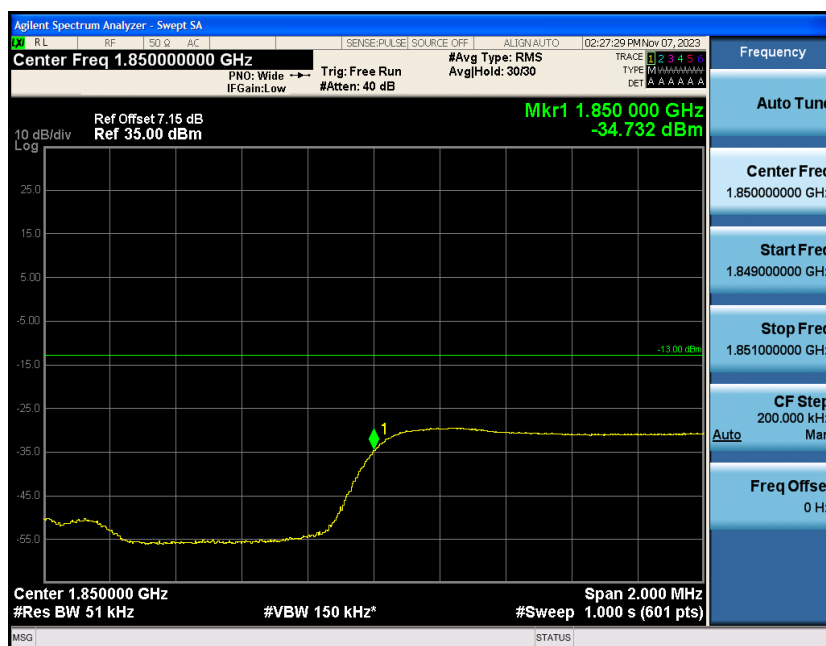
Band2-3MHz-QPSK-18615-15RB#0
