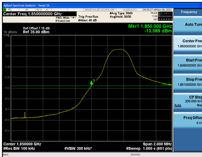
Band2-5MHz-QPSK-18625-1RB#24
