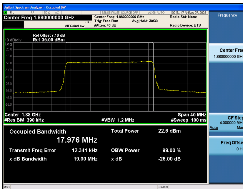
Band2-20MHz-QPSK-19100-100RB#0
