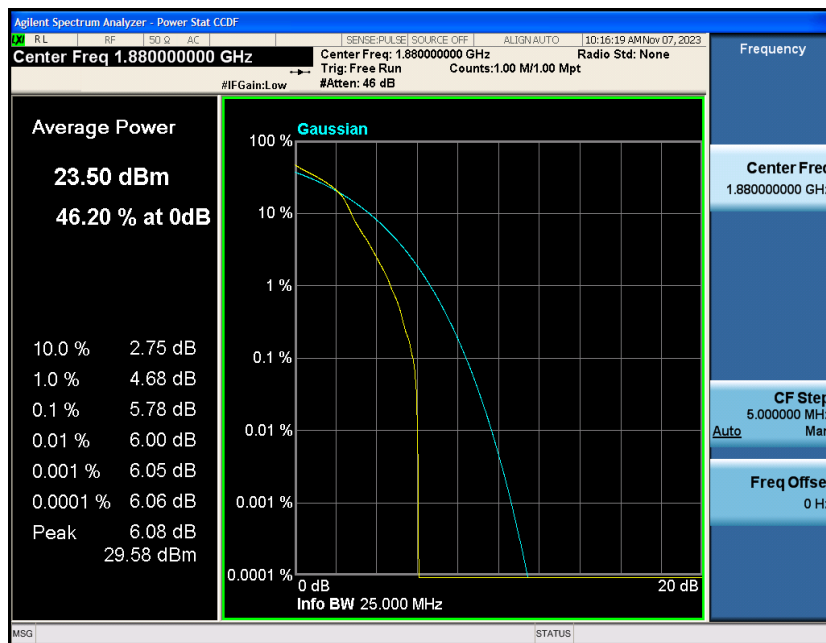
Band2-10MHz-16QAM-18900-50RB#0
