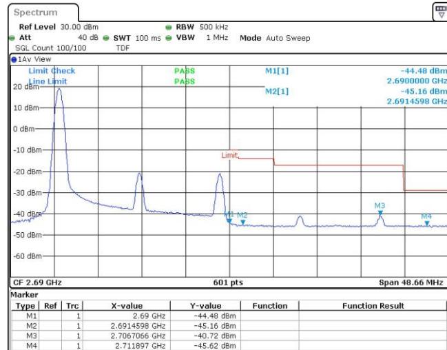
Band41-20MHz-16QAM-41490-1RB#99
