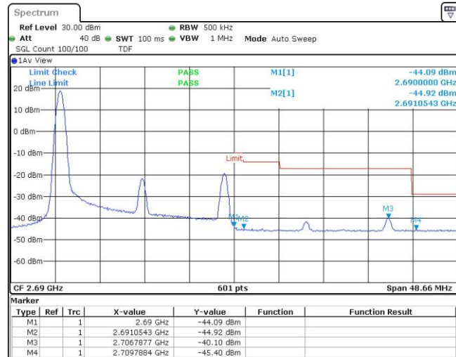
Band41-20MHz-QPSK-41490-1RB#99
