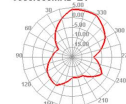
6000.000MHz E1
