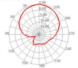
5550.000MHz E2
