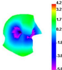
2450.000MHz E1
