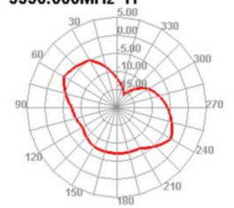
5550.000MHz E2
