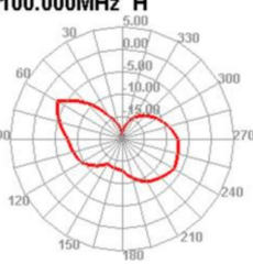
5100.000MHz H
