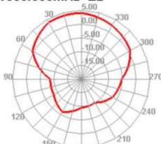
6000.000MHz E2
