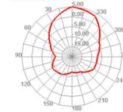
5550.000MHz E1
