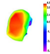
6000.000MHz E1
