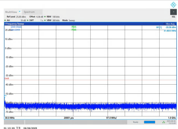
NTNV-n7-PC3-15-25-M-DFT-QPSK-Edge_1RB_Left-30-1000-PA SS
