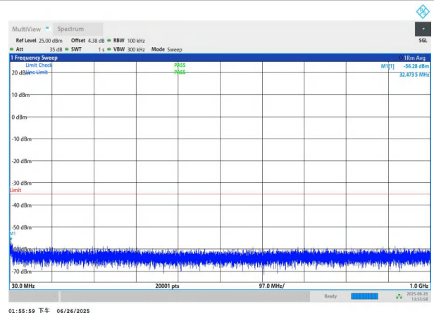
NTNV-n7-PC3-15-30-M-DFT-QPSK-Edge_1RB_Left-30-1000-PA SS
