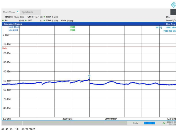
NTNV-n66-PC3-15-20-L-DFT-BPSK-Edge_1RB_Left-3000-12000 -PASS
