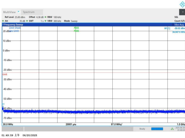
NTNV-n66-PC3-15-20-H-DFT-BPSK-Edge_1RB_Left-30-1000-P ASS
