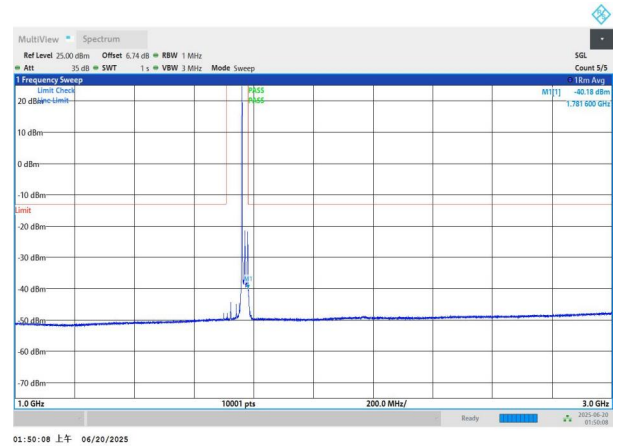
NTNV-n66-PC3-15-20-H-DFT-BPSK-Edge_1RB_Left-1000-3000-P ASS
