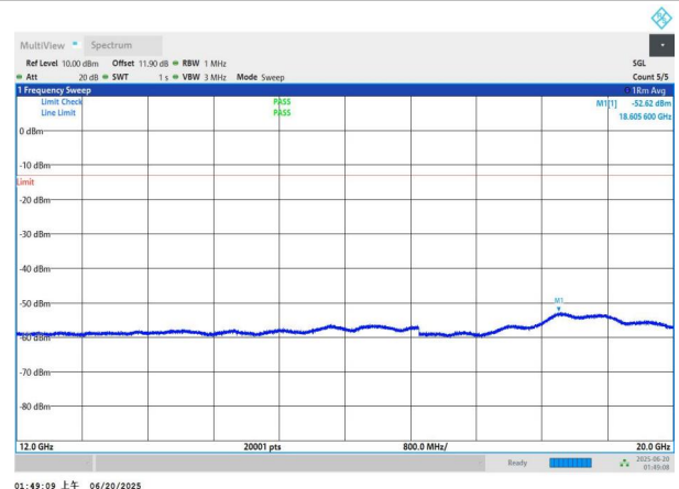
NTNV-n66-PC3-15-20-M-DFT-QPSK-Edge_1RB_Left-12000-2000 0-PASS
