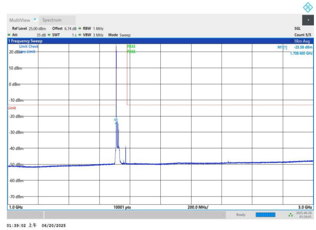
NTNV-n66-PC3-15-15-L-DFT-QPSK-Edge_1RB_Left-1000-3000-P ASS
