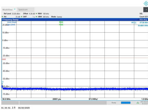
NTNV-n66-PC3-15-10-M-DFT-QPSK-Edge_1RB_Left-30-1000-P ASS
