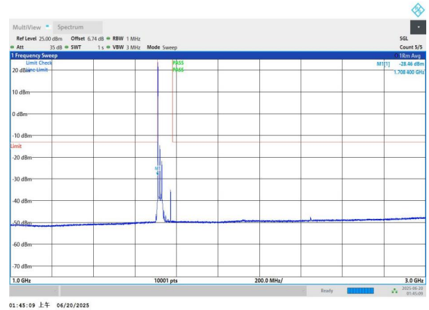
NTNV-n66-PC3-15-20-L-DFT-BPSK-Edge_1RB_Left-1000-3000-P ASS
