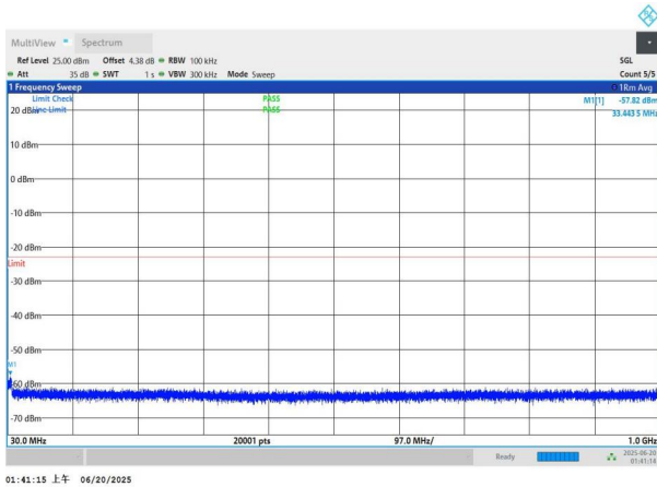
NTNV-n66-PC3-15-15-M-DFT-QPSK-Edge_1RB_Left-30-1000-P ASS
