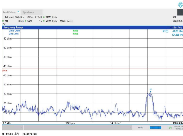
NTNV-n66-PC3-15-15-M-DFT-QPSK-Edge_1RB_Left-0.009-0.15 -PASS
