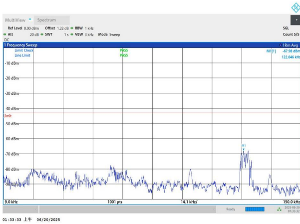
NTNV-n66-PC3-15-10-M-DFT-QPSK-Edge_1RB_Left-0.009-0.15 -PASS
