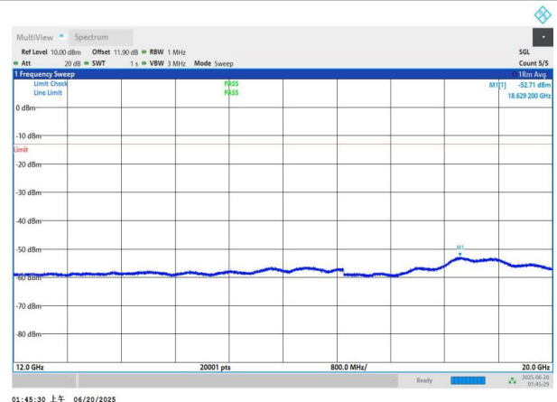
NTNV-n66-PC3-15-20-L-DFT-BPSK-Edge_1RB_Left-12000-20000 -PASS
