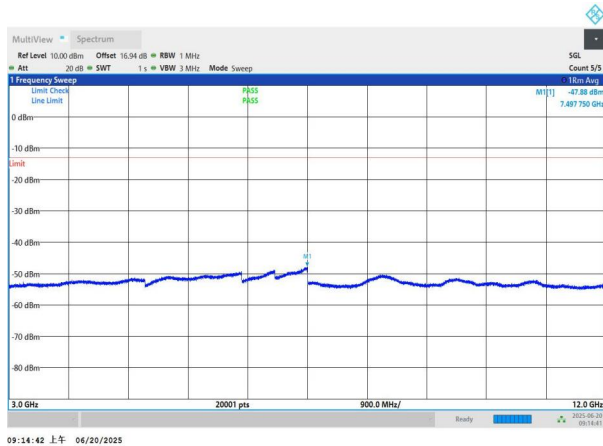
NTNV-n26(824-849)-PC3-15-20-M-DFT-QPSK-Edge_1RB_Left-3 000-12000-PASS
