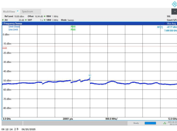
NTNV-n26(824-849)-PC3-15-20-L-DFT-QPSK-Edge_1RB_Left-3 000-12000-PASS
