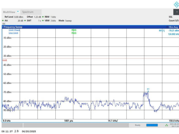
NTNV-n26(824-849)-PC3-15-20-L-DFT-QPSK-Edge_1RB_Left-0. 009-0.15-PASS
