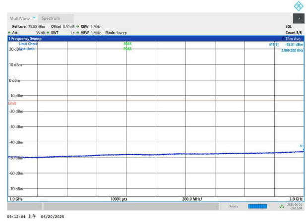
NTNV-n26(824-849)-PC3-15-20-L-DFT-QPSK-Edge_1RB_Left-10 00-3000-PASS
