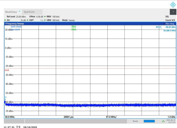
NTNV-n77(3450-3550)-PC3-30-60-M-DFT-QPSK-Edge_1RB_Left -30-1000-PASS
