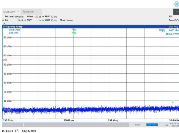
NTNV-n77(3450-3550)-PC3-30-60-L-DFT-QPSK-Edge_1RB_Left- 0.15-30-PASS
