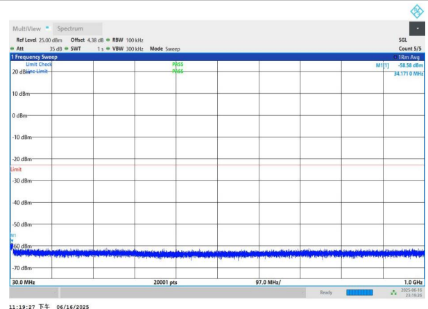
NTNV-n77(3450-3550)-PC3-30-50-M-DFT-QPSK-Edge_1RB_Left -30-1000-PASS
