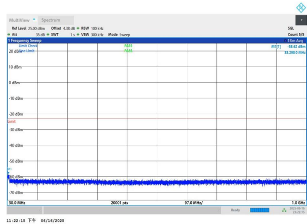
NTNV-n77(3450-3550)-PC3-30-50-H-DFT-QPSK-Edge_1RB_Left -30-1000-PASS
