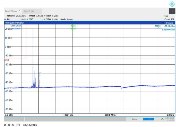
NTNV-n77(3450-3550)-PC3-30-50-H-DFT-QPSK-Edge_1RB_Left -3000-6000-PASS
