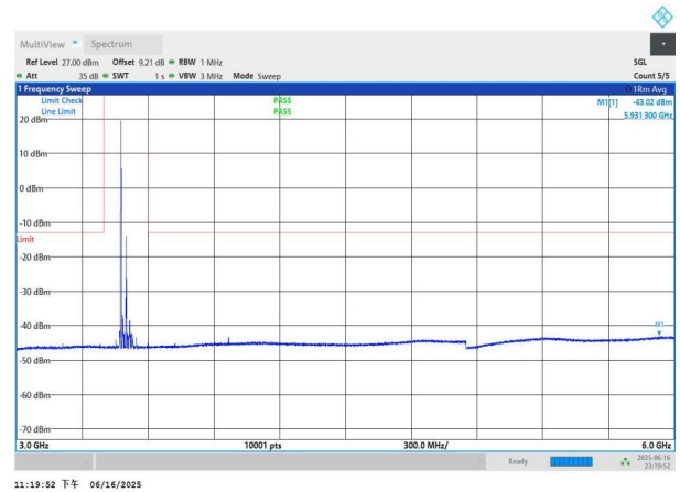
NTNV-n77(3450-3550)-PC3-30-50-M-DFT-QPSK-Edge_1RB_Left -3000-6000-PASS
