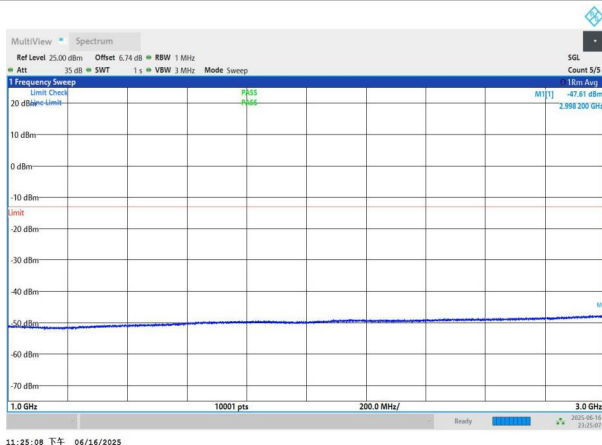
NTNV-n77(3450-3550)-PC3-30-60-L-DFT-QPSK-Edge_1RB_Left- 1000-3000-PASS
