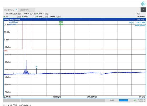
NTNV-n77(3450-3550)-PC3-30-60-L-DFT-QPSK-Edge_1RB_Left- 3000-6000-PASS
