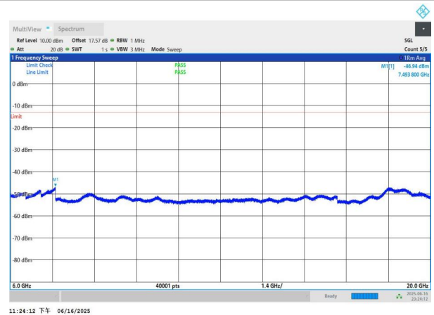
NTNV-n77(3450-3550)-PC3-30-60-L-DFT-BPSK-Edge_1RB_Left- 6000-20000-PASS
