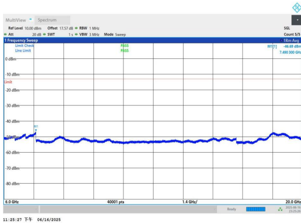
NTNV-n77(3450-3550)-PC3-30-60-L-DFT-QPSK-Edge_1RB_Left- 6000-20000-PASS
