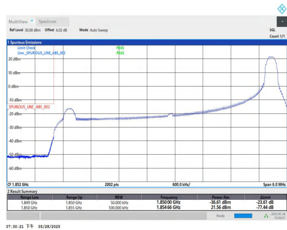
Band2-5MHz-QPSK-18625-1RB#24-PASS
