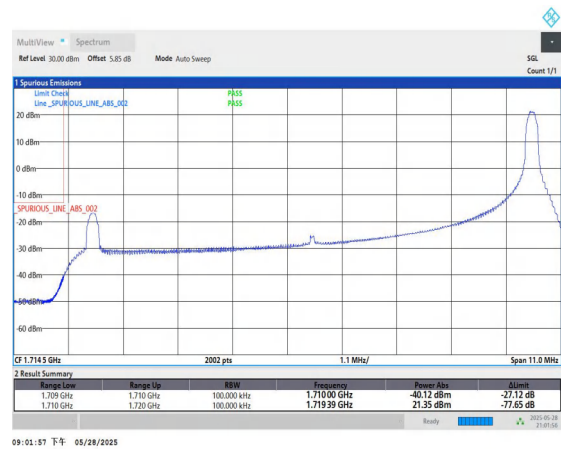
Band4-10MHz-QPSK-20000-1RB#49-PASS
