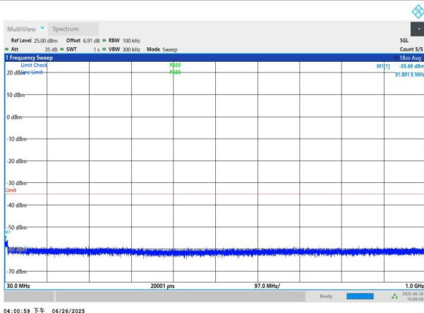
NTNV-n41-PC3-30-30-H-DFT-BPSK-Edge_1RB_Left-30-1000-P ASS
