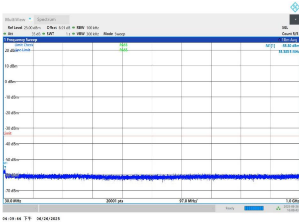
NTNV-n41-PC3-30-50-M-DFT-BPSK-Edge_1RB_Left-30-1000-P ASS
