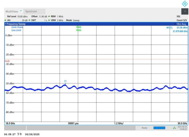
NTNV-n41-PC3-30-50-L-DFT-BPSK-Edge_1RB_Left-18000-3000
