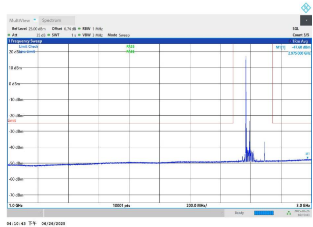
NTNV-n41-PC3-30-50-M-DFT-QPSK-Edge_1RB_Left-1000-3000- PASS
