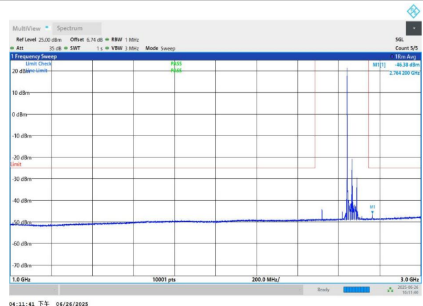
NTNV-n41-PC3-30-50-H-DFT-BPSK-Edge_1RB_Left-1000-3000-P ASS
