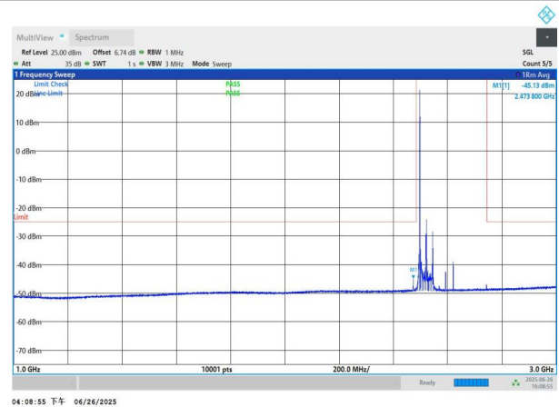
NTNV-n41-PC3-30-50-L-DFT-QPSK-Edge_1RB_Left-1000-3000-P
