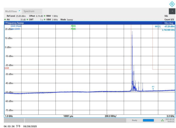
NTNV-n41-PC3-30-40-L-DFT-QPSK-Edge_1RB_Left-1000-3000-P ASS
