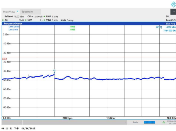
NTNV-n41-PC3-30-50-H-DFT-BPSK-Edge_1RB_Left-3000-1800 0-PASS
