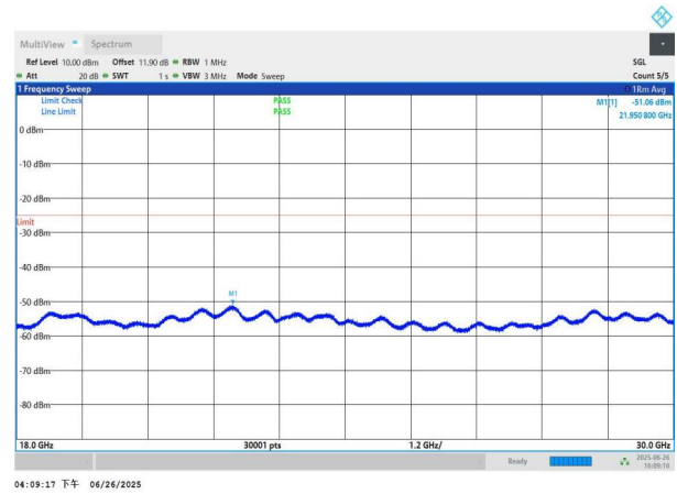
NTNV-n41-PC3-30-50-L-DFT-QPSK-Edge_1RB_Left-18000-3000 0-PASS
