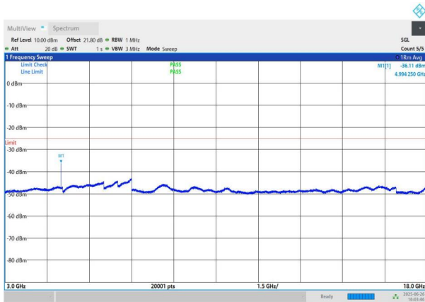
NTNV-n41-PC3-30-40-L-DFT-QPSK-Edge_1RB_Left-3000-1800 0-PASS
