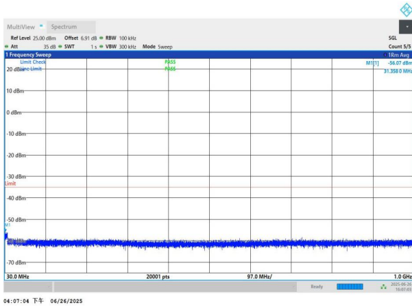
NTNV-n41-PC3-30-40-H-DFT-QPSK-Edge_1RB_Left-30-1000-P ASS
