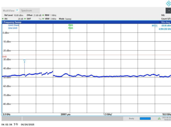
NTNV-n41-PC3-30-40-L-DFT-BPSK-Edge_1RB_Left-3000-18000 -PASS
