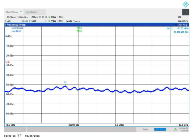
NTNV-n41-PC3-30-30-M-DFT-QPSK-Edge_1RB_Left-18000-3000 0-PASS
