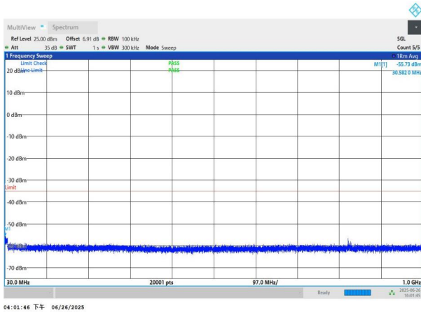
NTNV-n41-PC3-30-30-H-DFT-QPSK-Edge_1RB_Left-30-1000-P ASS
