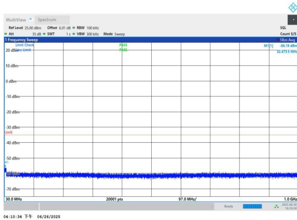
NTNV-n41-PC3-30-50-M-DFT-QPSK-Edge_1RB_Left-30-1000-P ASS
