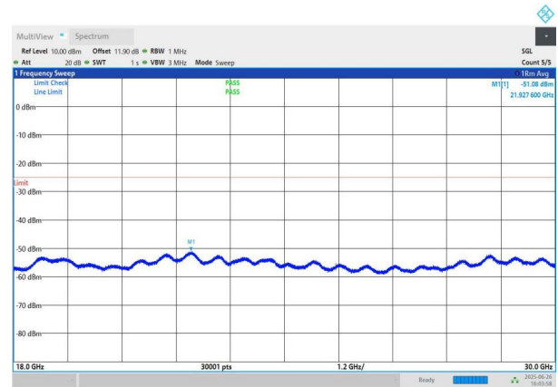
NTNV-n41-PC3-30-40-L-DFT-QPSK-Edge_1RB_Left-18000-3000 0-PASS
