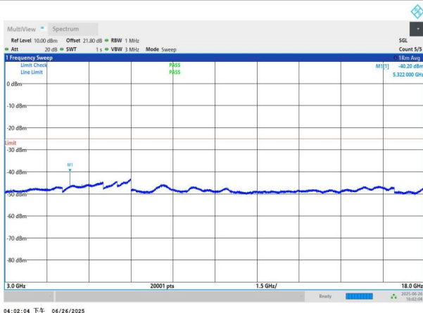
NTNV-n41-PC3-30-30-H-DFT-QPSK-Edge_1RB_Left-3000-1800 0-PASS
