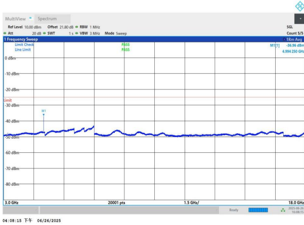
NTNV-n41-PC3-30-50-L-DFT-BPSK-Edge_1RB_Left-3000-18000
