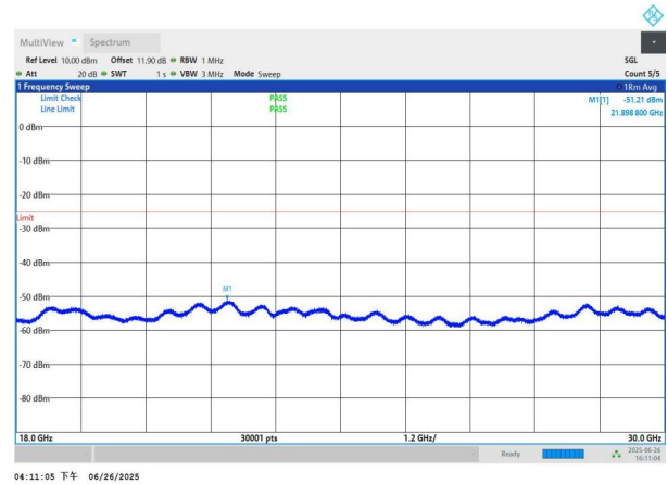
NTNV-n41-PC3-30-50-M-DFT-QPSK-Edge_1RB_Left-18000-3000 0-PASS
