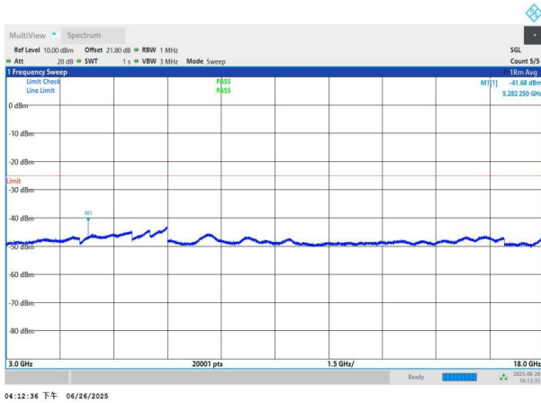
NTNV-n41-PC3-30-50-H-DFT-QPSK-Edge_1RB_Left-3000-1800 0-PASS
