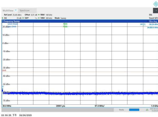
NTNV-n41-PC3-30-30-M-DFT-QPSK-Edge_1RB_Left-30-1000-P ASS
