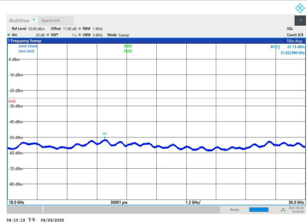
NTNV-n41-PC3-30-50-M-DFT-BPSK-Edge_1RB_Left-18000-3000 0-PASS
