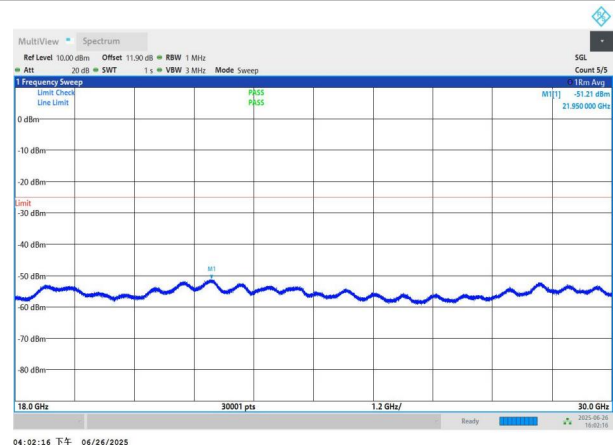
NTNV-n41-PC3-30-30-H-DFT-QPSK-Edge_1RB_Left-18000-3000 0-PASS
