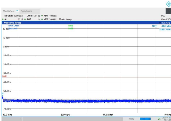
NTNV-n41-PC3-30-40-M-DFT-BPSK-Edge_1RB_Left-30-1000-P ASS
