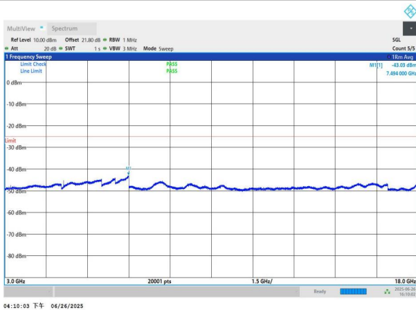
NTNV-n41-PC3-30-50-M-DFT-BPSK-Edge_1RB_Left-3000-1800 0-PASS
