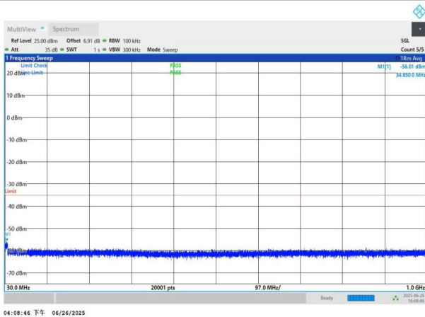
NTNV-n41-PC3-30-50-L-DFT-QPSK-Edge_1RB_Left-30-1000-PA
