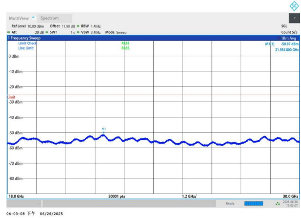
NTNV-n41-PC3-30-40-L-DFT-BPSK-Edge_1RB_Left-18000-3000 0-PASS
