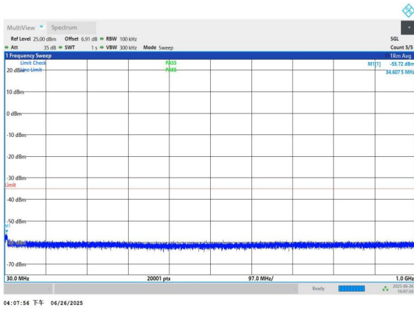
NTNV-n41-PC3-30-50-L-DFT-BPSK-Edge_1RB_Left-30-1000-PA
