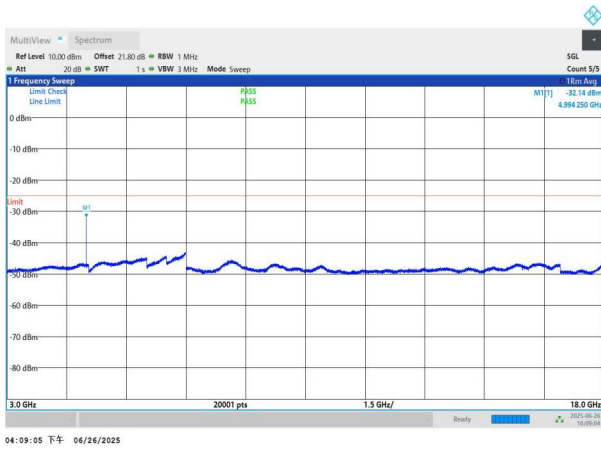
NTNV-n41-PC3-30-50-L-DFT-QPSK-Edge_1RB_Left-3000-1800 0-PASS
