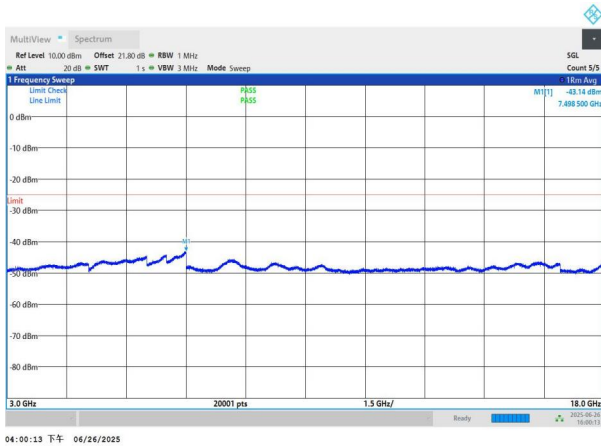
NTNV-n41-PC3-30-30-M-DFT-QPSK-Edge_1RB_Left-3000-1800 0-PASS
