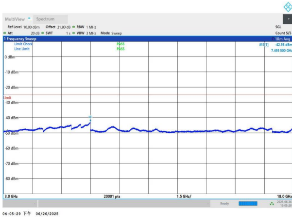
NTNV-n41-PC3-30-40-M-DFT-QPSK-Edge_1RB_Left-3000-1800 0-PASS
