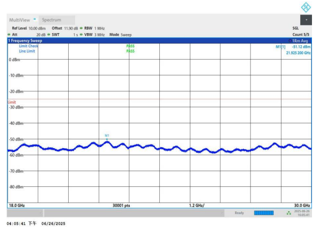
NTNV-n41-PC3-30-40-M-DFT-QPSK-Edge_1RB_Left-18000-3000 0-PASS
