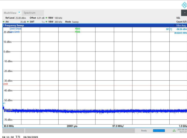
NTNV-n41-PC3-30-50-H-DFT-BPSK-Edge_1RB_Left-30-1000-P ASS
