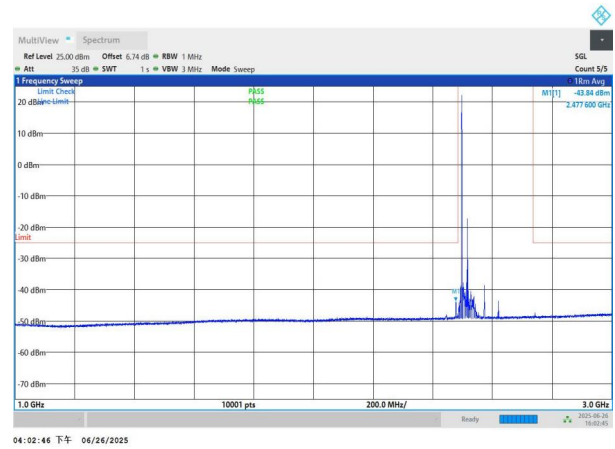
NTNV-n41-PC3-30-40-L-DFT-BPSK-Edge_1RB_Left-1000-3000-P ASS
