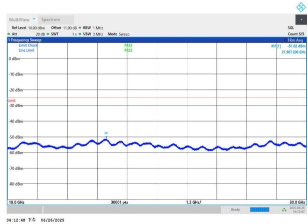
NTNV-n41-PC3-30-50-H-DFT-QPSK-Edge_1RB_Left-18000-3000 0-PASS
