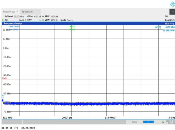
NTNV-n41-PC3-30-40-M-DFT-QPSK-Edge_1RB_Left-30-1000-P ASS
