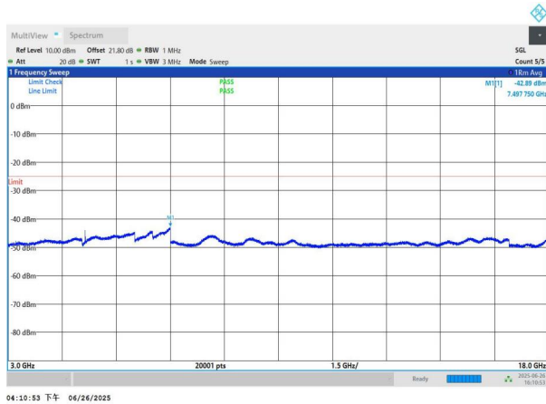
NTNV-n41-PC3-30-50-M-DFT-QPSK-Edge_1RB_Left-3000-1800 0-PASS
