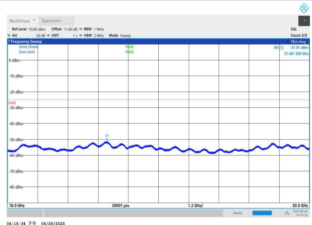
NTNV-n41-PC3-30-60-M-DFT-BPSK-Edge_1RB_Left-18000-3000 0-PASS
