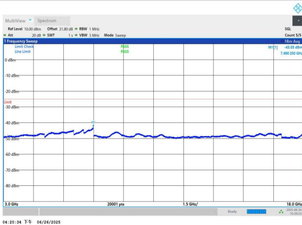
NTNV-n41-PC3-30-70-M-DFT-BPSK-Edge_1RB_Left-3000-1800 0-PASS
