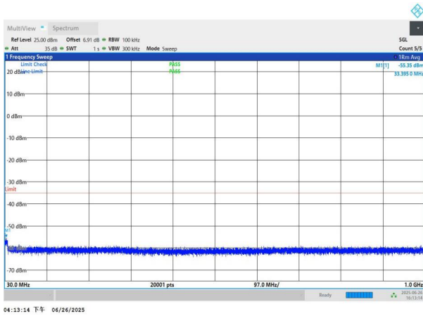
NTNV-n41-PC3-30-60-L-DFT-BPSK-Edge_1RB_Left-30-1000-PA SS
