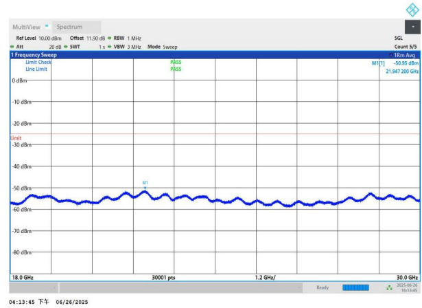
NTNV-n41-PC3-30-60-L-DFT-BPSK-Edge_1RB_Left-18000-3000 0-PASS
