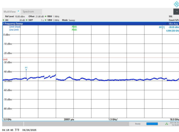
NTNV-n41-PC3-30-70-L-DFT-BPSK-Edge_1RB_Left-3000-18000
