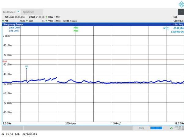
NTNV-n41-PC3-30-60-L-DFT-BPSK-Edge_1RB_Left-3000-18000 -PASS
