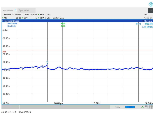
NTNV-n41-PC3-30-60-M-DFT-BPSK-Edge_1RB_Left-3000-1800 0-PASS
