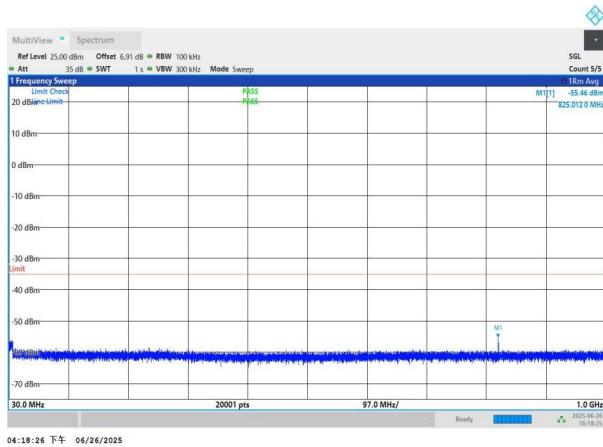
NTNV-n41-PC3-30-70-L-DFT-BPSK-Edge_1RB_Left-30-1000-PA
