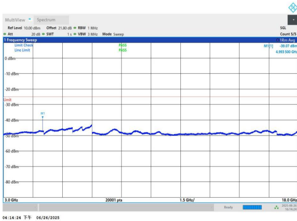
NTNV-n41-PC3-30-60-L-DFT-QPSK-Edge_1RB_Left-3000-1800 0-PASS
