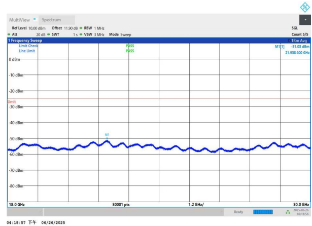
NTNV-n41-PC3-30-70-L-DFT-BPSK-Edge_1RB_Left-18000-3000
