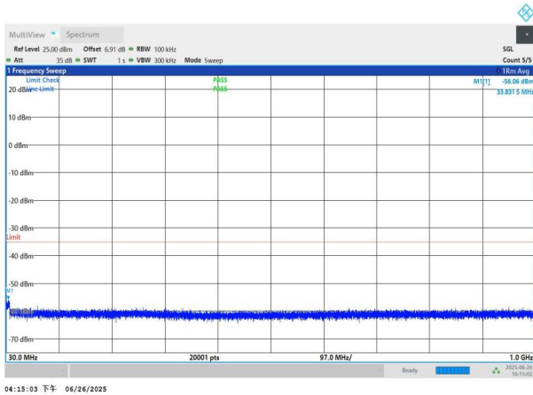
NTNV-n41-PC3-30-60-M-DFT-BPSK-Edge_1RB_Left-30-1000-P ASS
