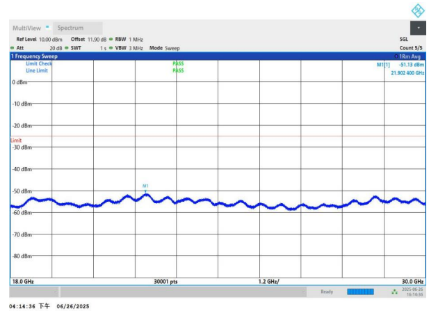
NTNV-n41-PC3-30-60-L-DFT-QPSK-Edge_1RB_Left-18000-3000 0-PASS
