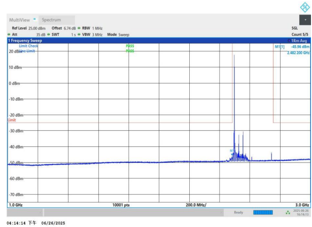
NTNV-n41-PC3-30-60-L-DFT-QPSK-Edge_1RB_Left-1000-3000-P ASS
