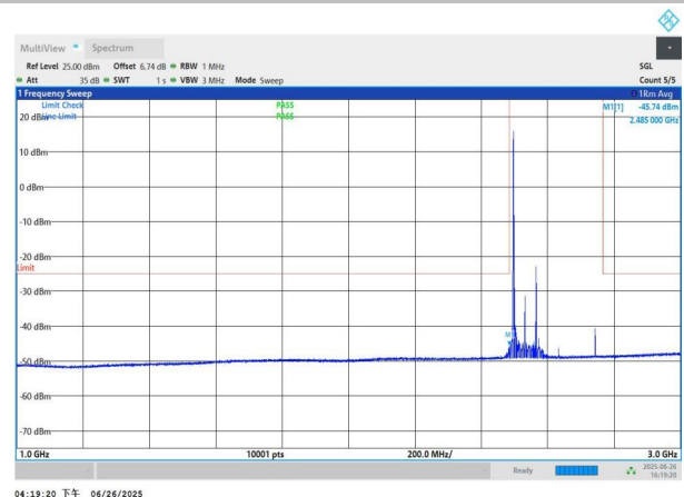
NTNV-n41-PC3-30-70-L-DFT-QPSK-Edge_1RB_Left-1000-3000-P
