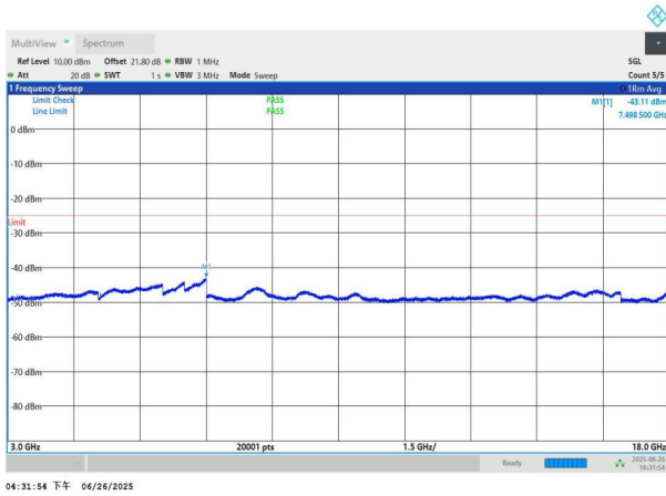
NTNV-n41-PC3-30-90-M-DFT-QPSK-Edge_1RB_Left-3000-1800 0-PASS
