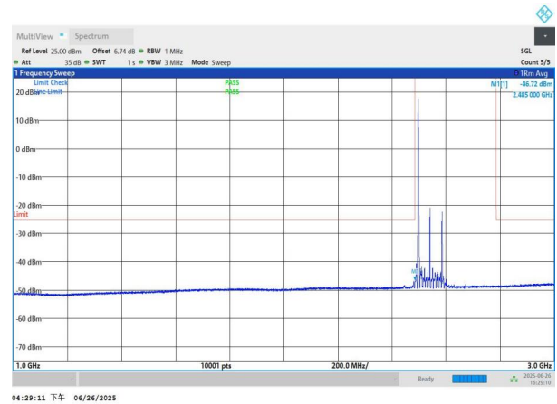
NTNV-n41-PC3-30-90-L-DFT-BPSK-Edge_1RB_Left-1000-3000-P ASS
