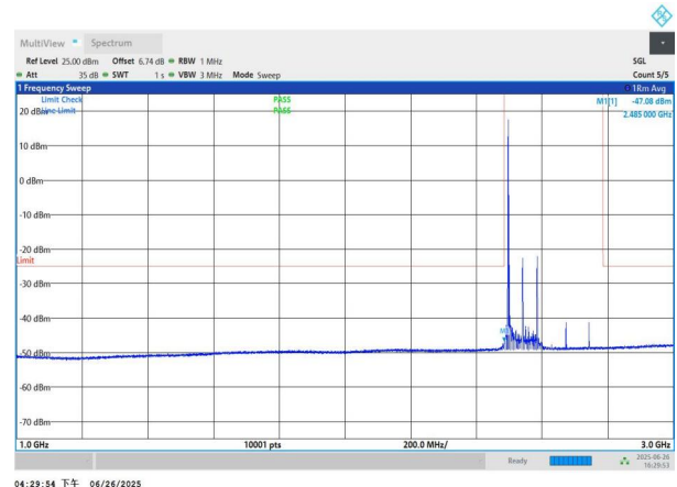
NTNV-n41-PC3-30-90-L-DFT-QPSK-Edge_1RB_Left-1000-3000-P ASS
