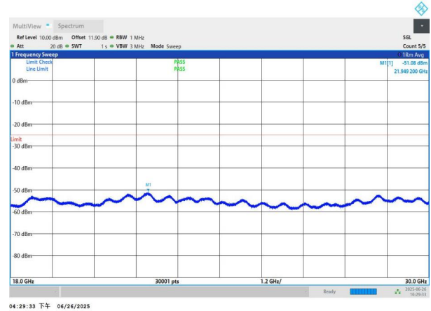
NTNV-n41-PC3-30-90-L-DFT-BPSK-Edge_1RB_Left-18000-3000 0-PASS
