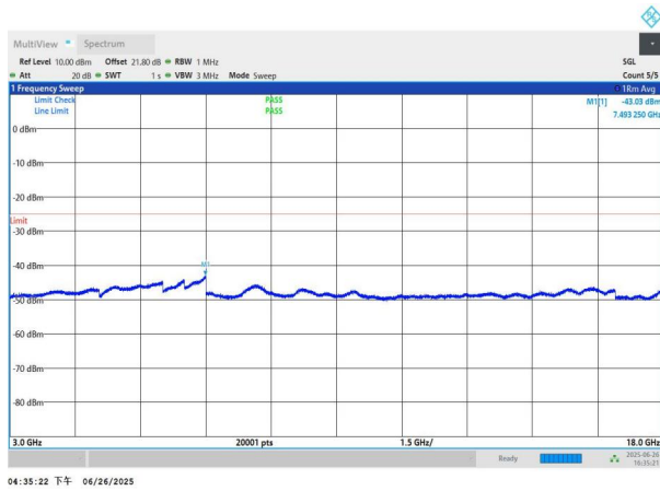
NTNV-n41-PC3-30-100-L-DFT-QPSK-Edge_1RB_Left-3000-180 00-PASS
