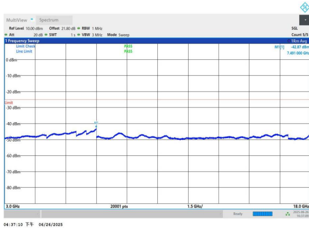
NTNV-n41-PC3-30-100-M-DFT-QPSK-Edge_1RB_Left-3000-18000-PASS
