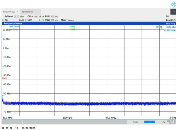
NTNV-n41-PC3-30-90-L-DFT-BPSK-Edge_1RB_Left-30-1000-PA SS
