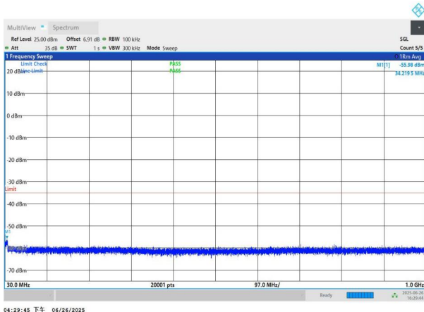
NTNV-n41-PC3-30-90-L-DFT-QPSK-Edge_1RB_Left-30-1000-PA SS
