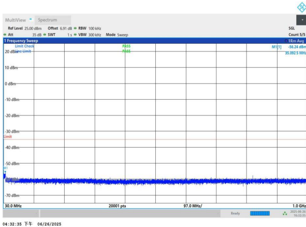
NTNV-n41-PC3-30-90-H-DFT-BPSK-Edge_1RB_Left-30-1000-P ASS
