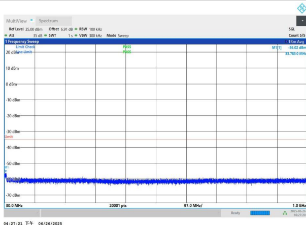
NTNV-n41-PC3-30-80-H-DFT-BPSK-Edge_1RB_Left-30-1000-P ASS
