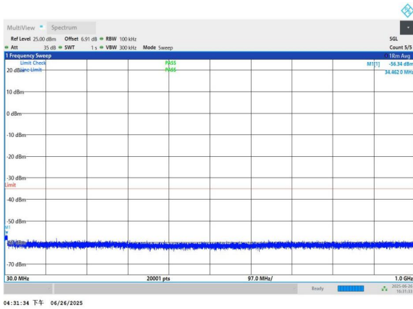
NTNV-n41-PC3-30-90-M-DFT-QPSK-Edge_1RB_Left-30-1000-P ASS
