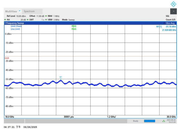
NTNV-n41-PC3-30-100-M-DFT-QPSK-Edge_1RB_Left-18000-30000-PASS
