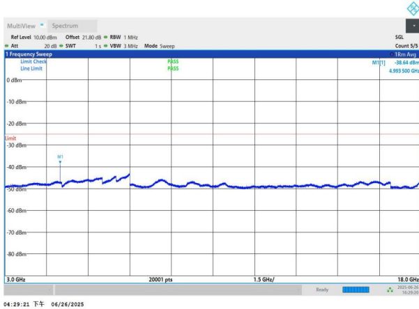
NTNV-n41-PC3-30-90-L-DFT-BPSK-Edge_1RB_Left-3000-18000 -PASS
