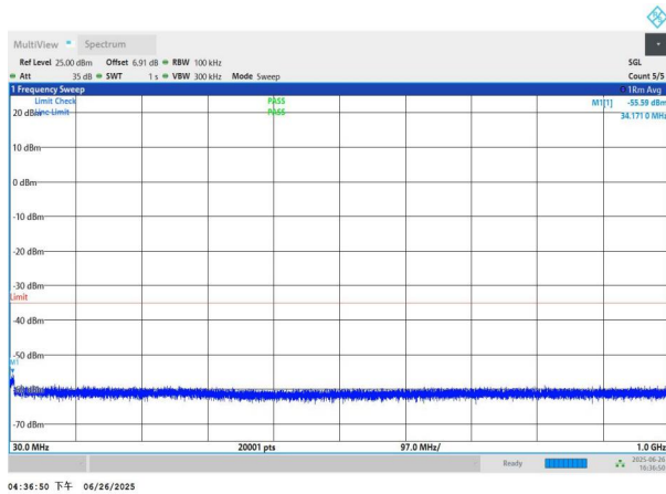
NTNV-n41-PC3-30-100-M-DFT-QPSK-Edge_1RB_Left-30-1000-PASS
