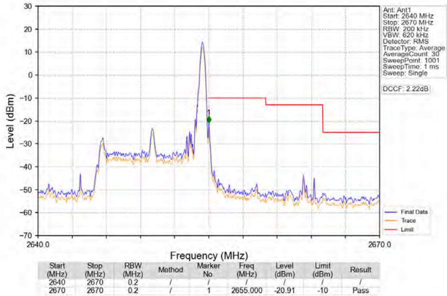
Band41_10MHz_16QAM_HCH_2650MHz_RB_1_49_NTNV
