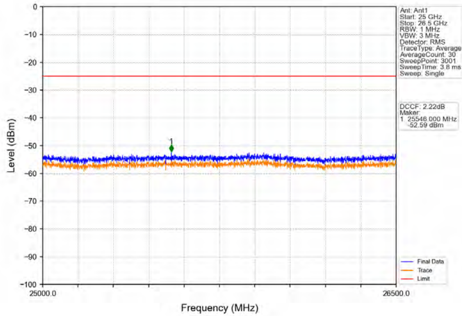
Band41_15MHz_QPSK_HCH_2647.5MHz_RB_1_74_NTNV
