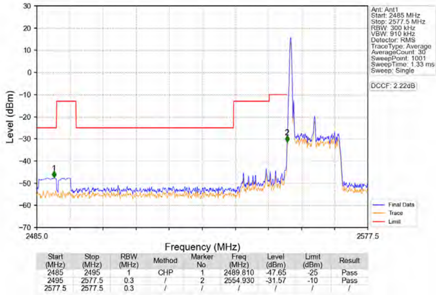
Band41_15MHz_QPSK_LCH_2562.5MHz_RB_1_0_NTNV
