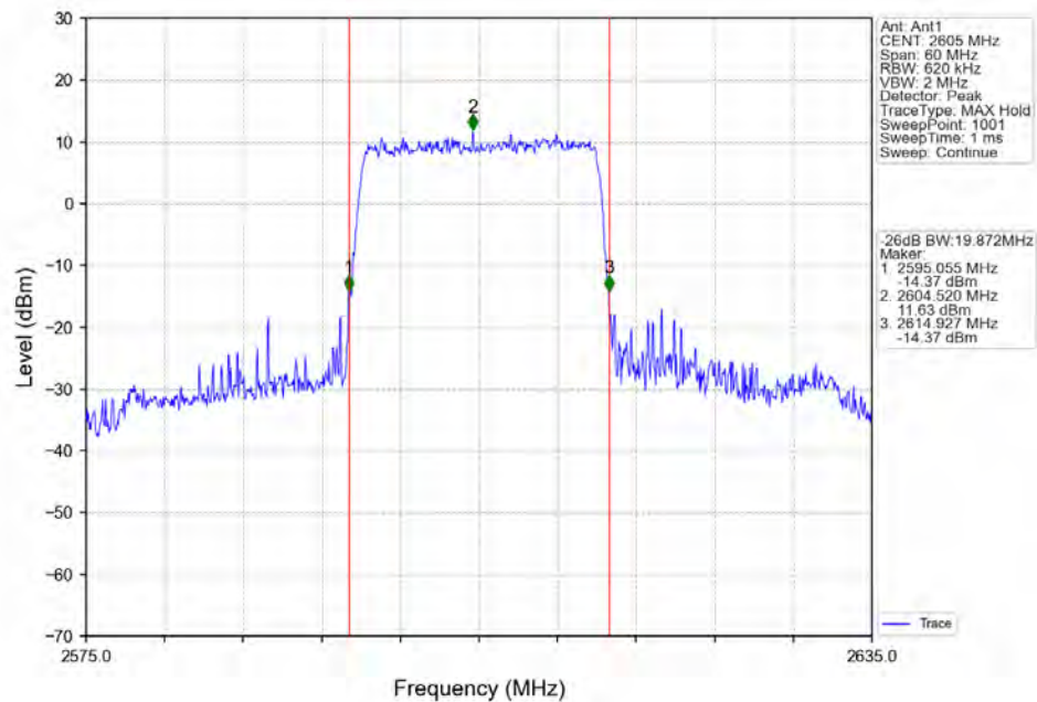
Band41_20MHz_QPSK_MCH_2605MHz_RB_100_0_NTNV
