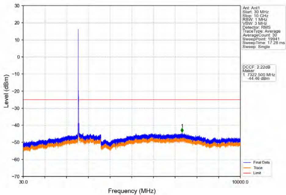
Band41 20MHz QPSK LCH 2565MHz RB 1 0 NTN
