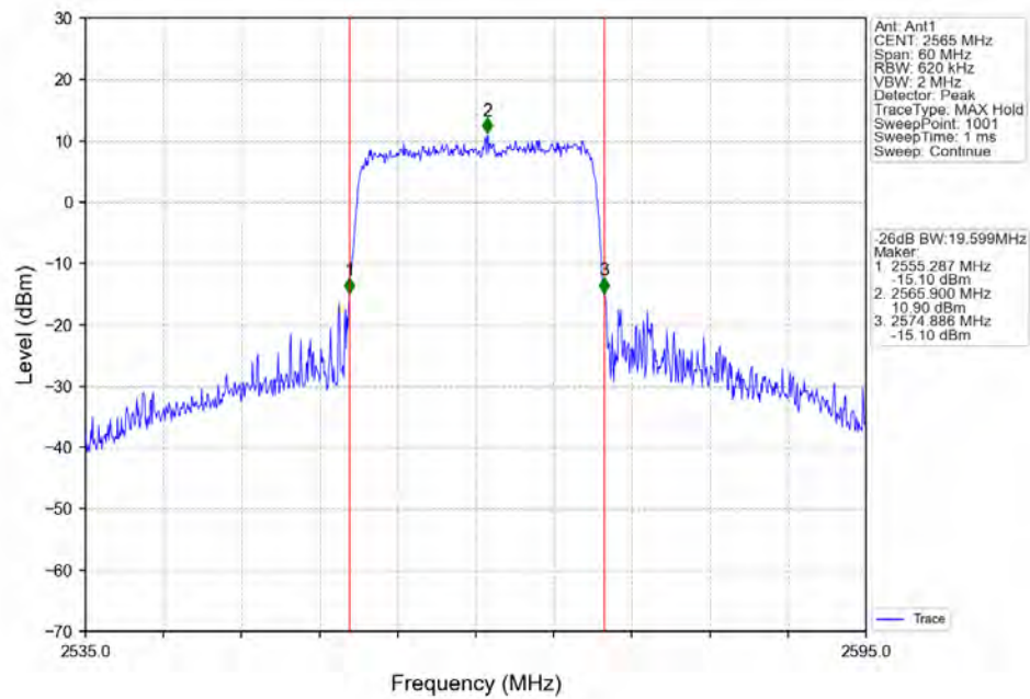
Band41_20MHz_16QAM_LCH_2565MHz_RB_100_0_NTNV
