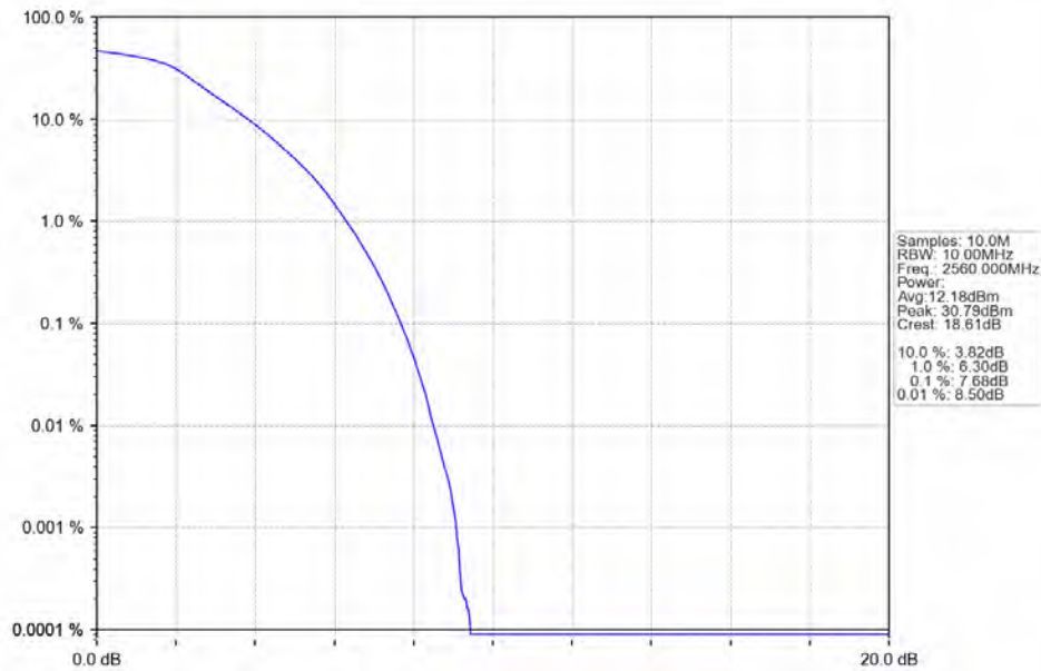
Band41 10MHz QPSK LCH 2560MHz RB 50 0 NTNV
