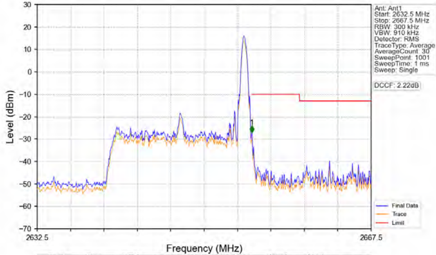
Band41_15MHz_QPSK_HCH_2647.5MHz_RB_1_74_NTNV
