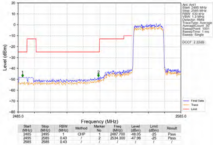
Band41_20MHz_QPSK_LCH_2565MHz_RB_100_0_NTNV
