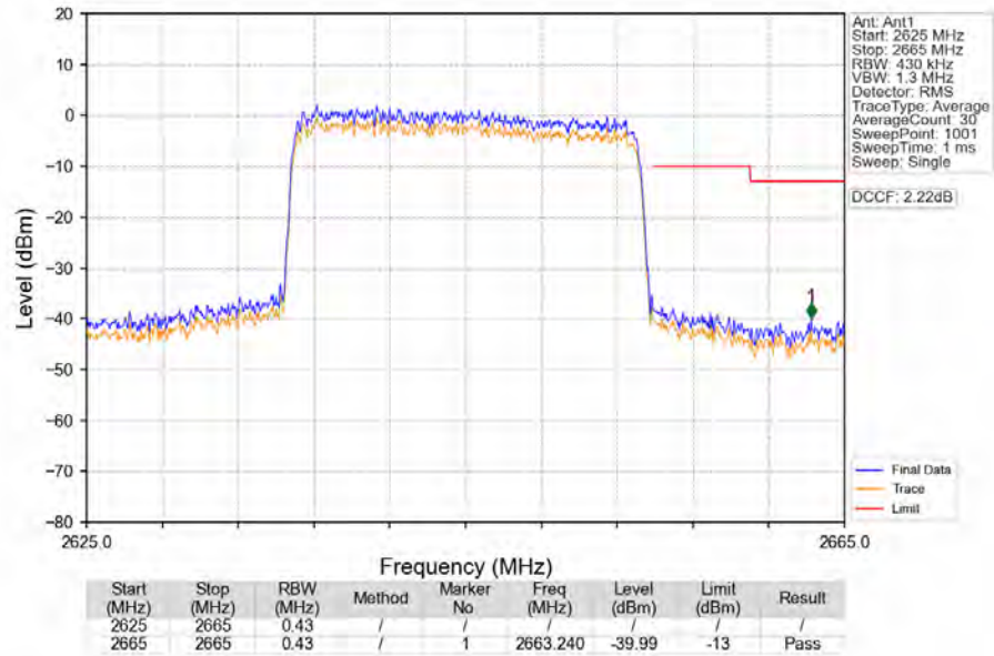
Band41_20MHz_QPSK_HCH_2645MHz_RB_100_0_NTNV
