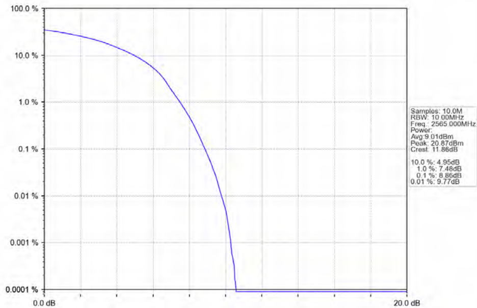
Band41_20MHz_16QAM_LCH_2565MHz_RB_100_0_NTNV
