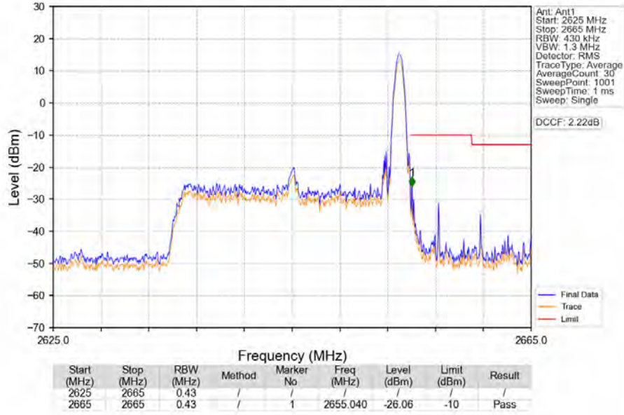
Band41_20MHz_QPSK_HCH_2645MHz_RB_1_99_NTNV
