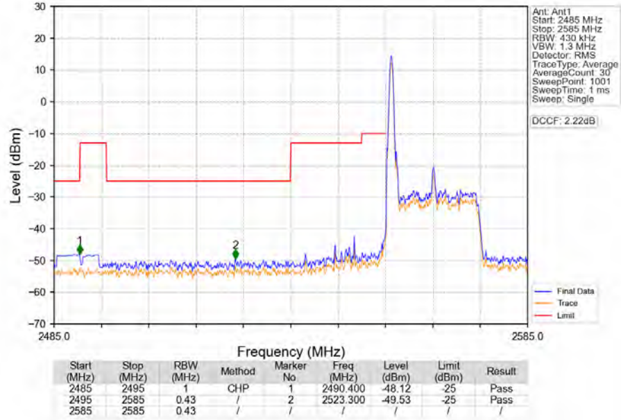
Band41_20MHz_16QAM_LCH_2565MHz_RB_1_0_NTNV
