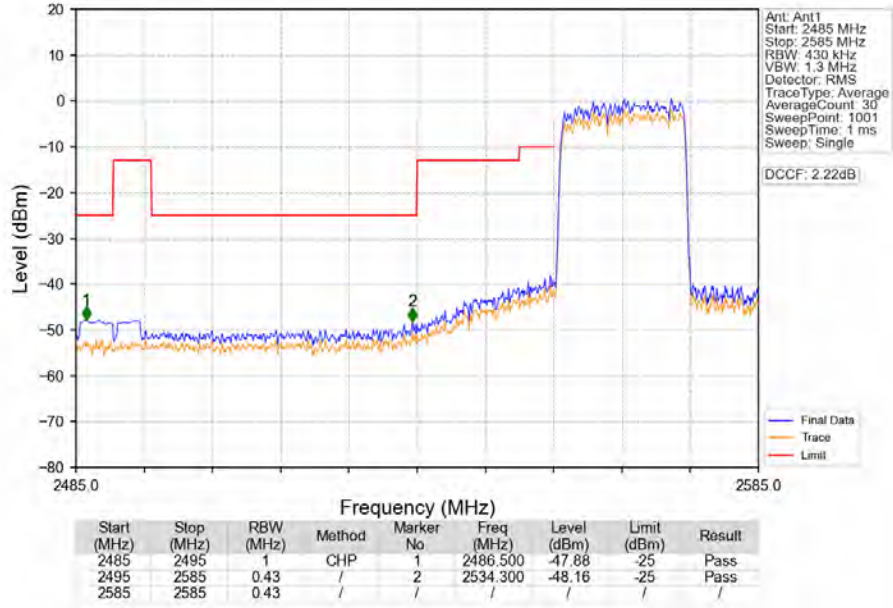
Band41_20MHz_16QAM_LCH_2565MHz_RB_100_0_NTNV
