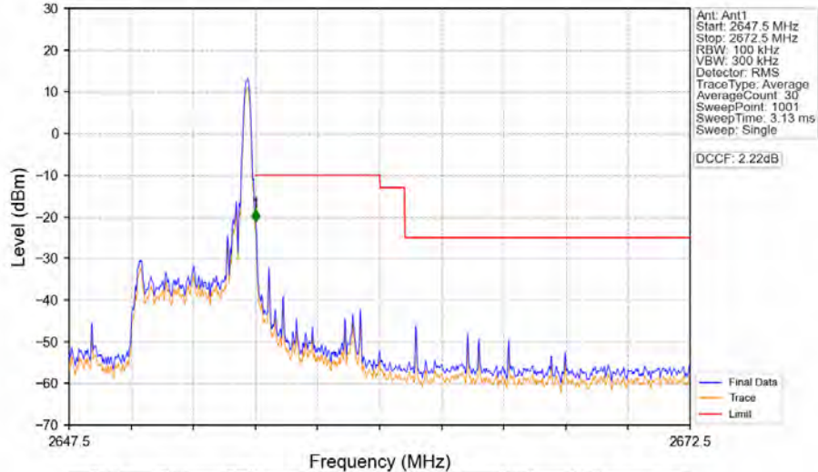
Band41_5MHz_QPSK_HCH_2652.5MHz_RB_1_24_NTNV
