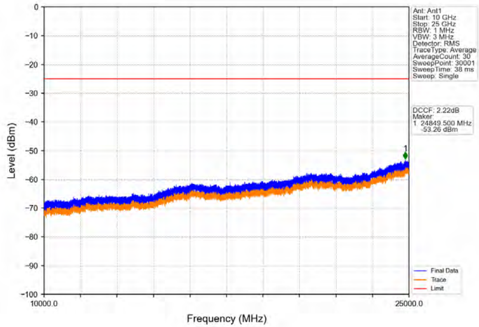
Band41_5MHz_QPSK_LCH_2557.5MHz_RB_1_0_NTNV
