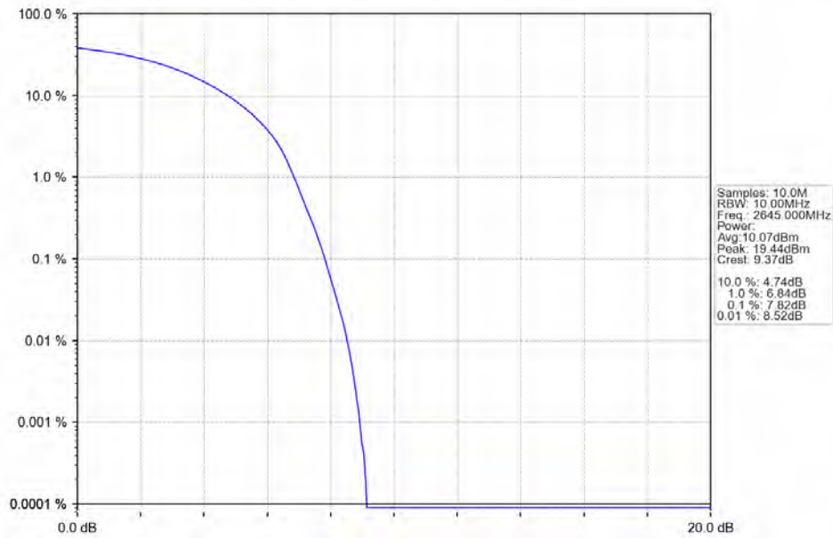
Band41_20MHz_QPSK_HCH_2645MHz_RB_100_0_NTNV
