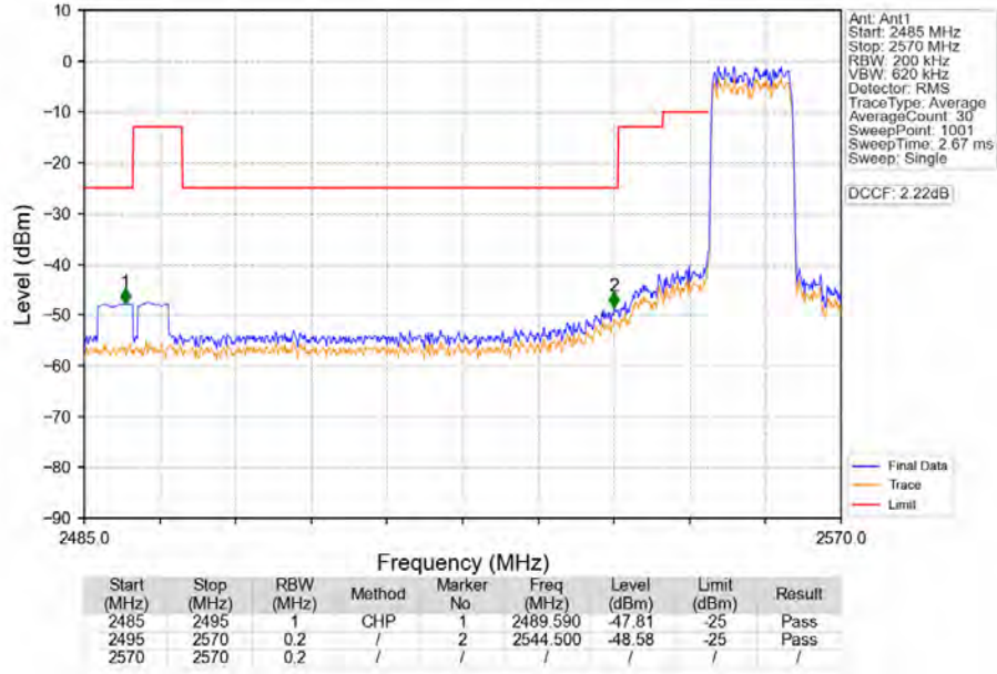
Band41_10MHz_16QAM_LCH_2560MHz_RB_50_0_NTNV
