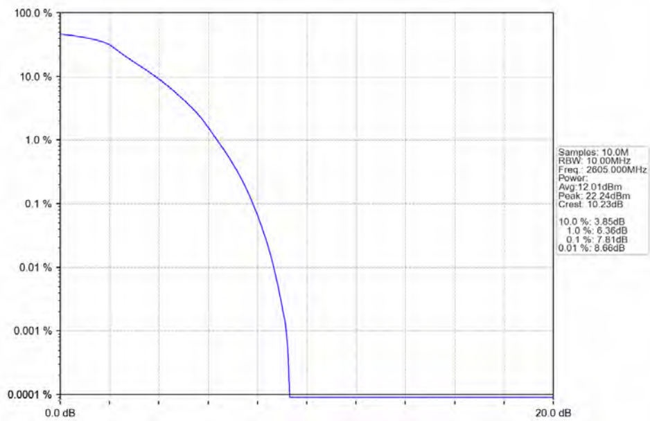
Band41 10MHz QPSK MCH 2605MHz RB 50 0 NTNV
