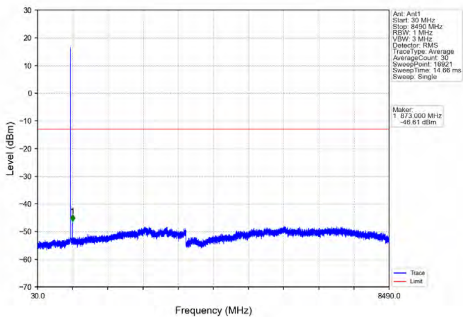
Band5 5MHz QPSK LCH 826.5MHz RB 1 0 NTV
