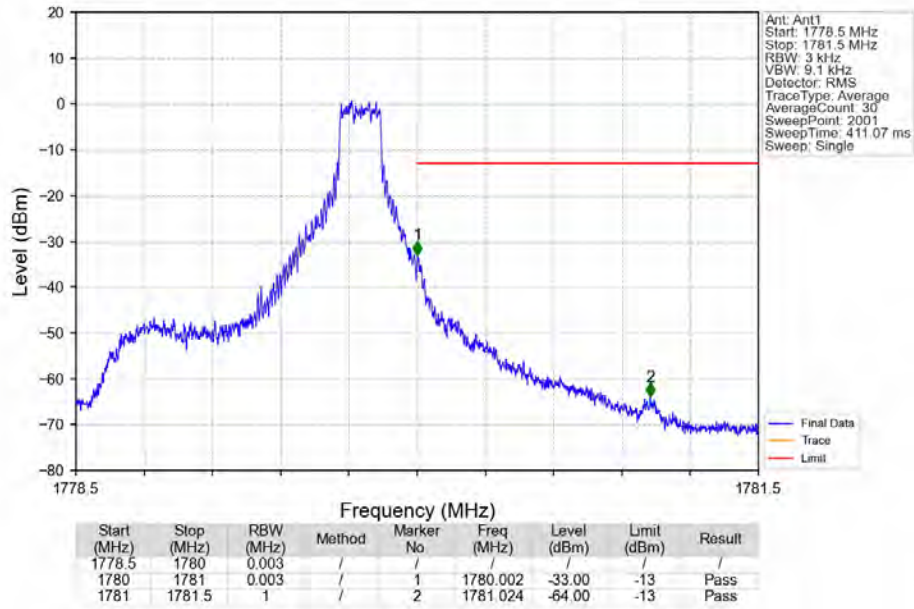
Band66 1.4MHz QPSK HCH 1779.3MHz RB 1 5 NTV
