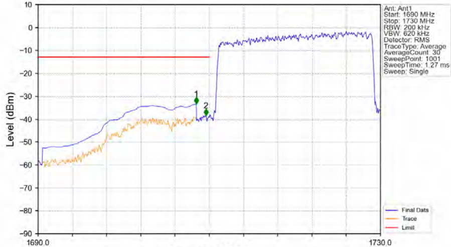
Band66_20MHz_16QAM_LCH_1720MHz_RB_100_0_NTNV
