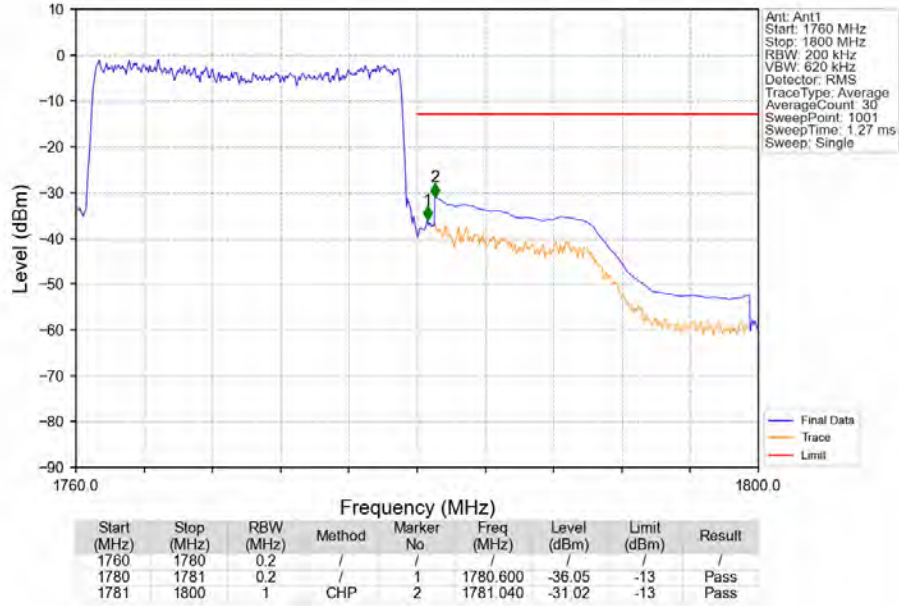
Band66_20MHz_QPSK_HCH_1770MHz_RB_100_0_NTNV
