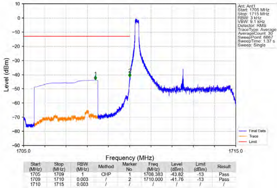
Band66 5MHz QPSK LCH 1712.5MHz RB 1 0 NTNV
