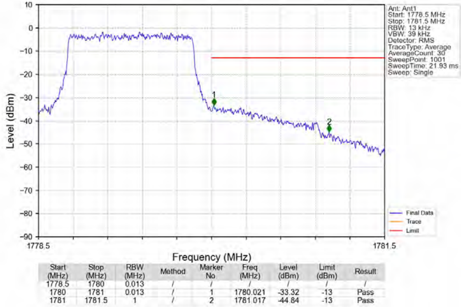
Band66 1.4MHz QPSK HCH 1779.3MHz RB 6 0 NTV
