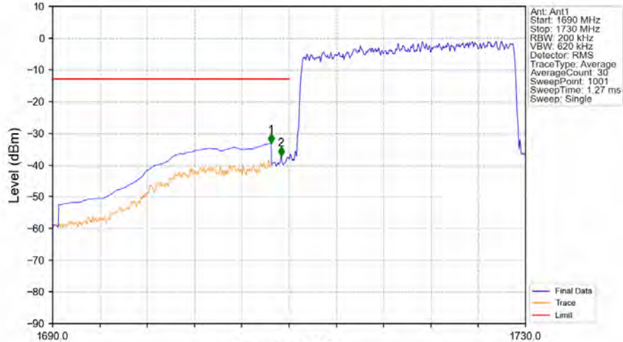
Band66_20MHz_QPSK_LCH_1720MHz_RB_100_0_NTNV
