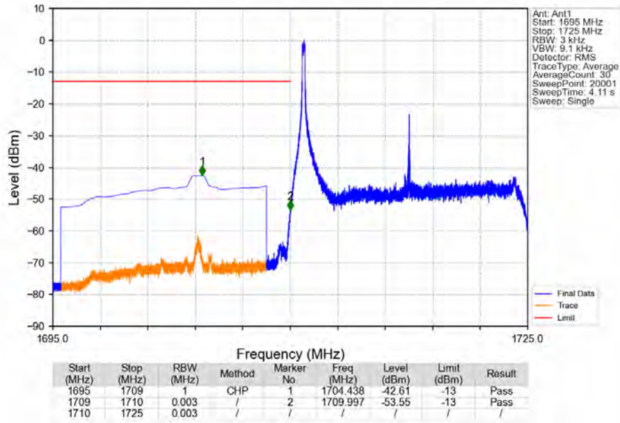
Band66 15MHz QPSK LCH 1717.5MHz RB 1 0 NTNV
