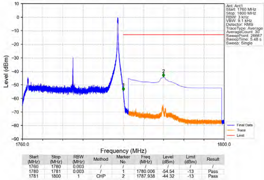
Band66_20MHz_16QAM_HCH_1770MHz_RB_1_99_NTNV
