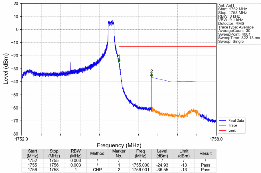
Band4_3MHz_QPSK_HCH_1753.5MHz_RB_1_14_NTNV
