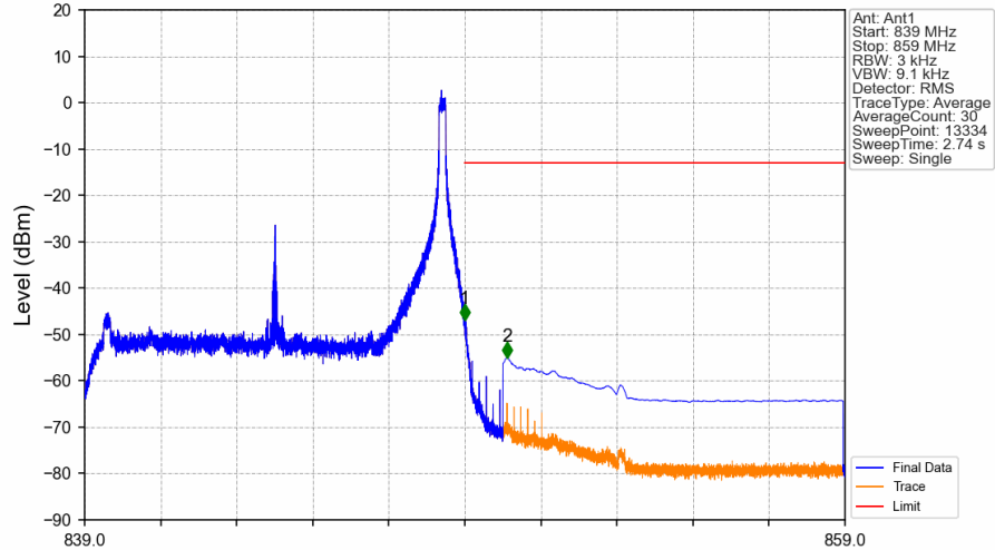
Band5_10MHz_QPSK_HCH_844MHz_RB_1_49_NTNV
