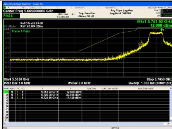
802.11(n20)-5745
