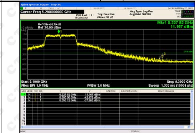
802.11n(HT40)-5230
