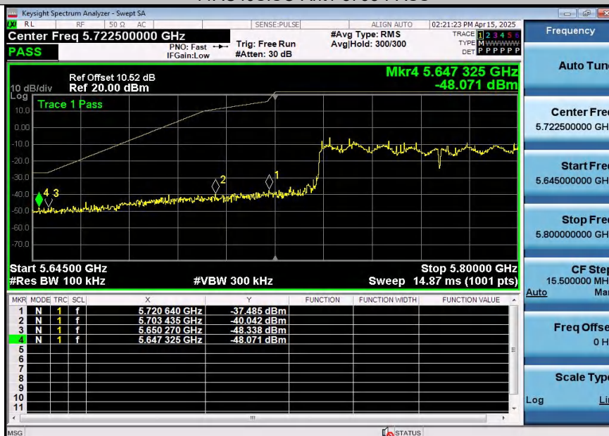
11AC80SISO-Ant1-5775-PASS
