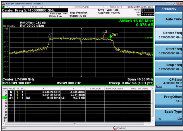
802.11ac(VHT20)
