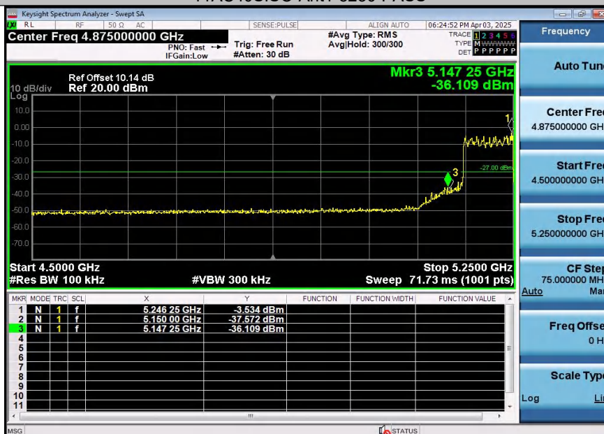
11AC80SISO-Ant1-5210-PASS
