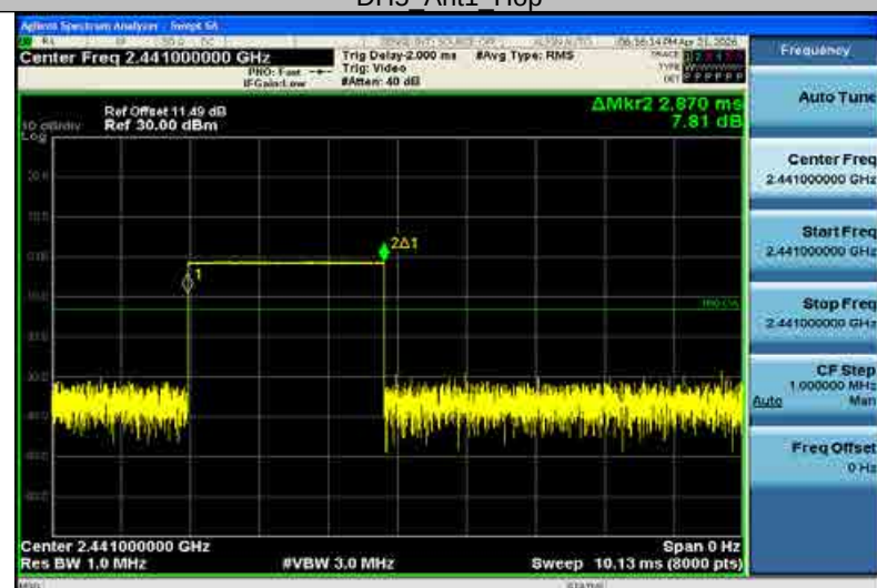
DH5_Ant1_Hop
