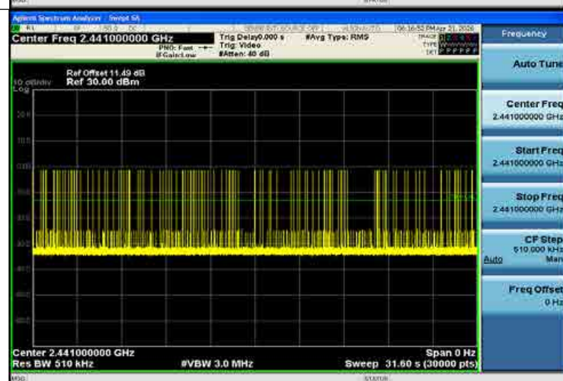
2DH1_Ant1_Hop
