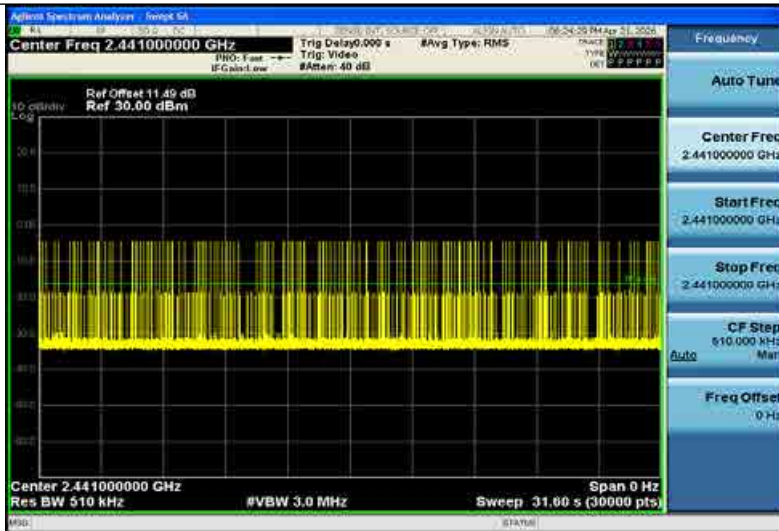
2DH5_Ant1_Hop
