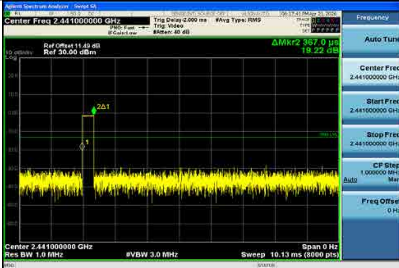
DH1_Ant1_Hop
