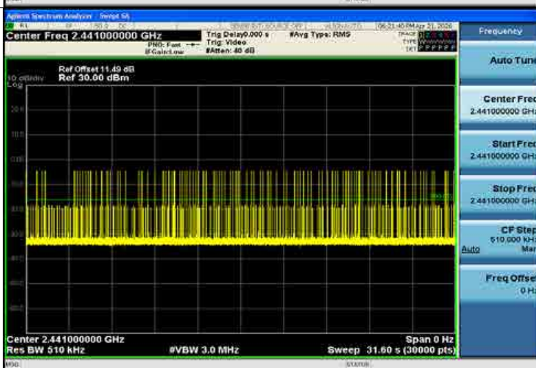
3DH1_Ant1_Hop
