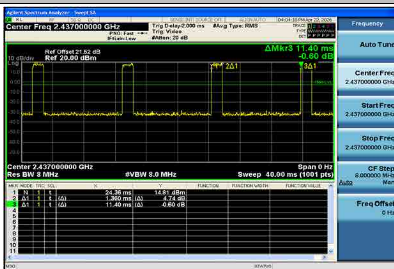
NTNV-11G-Ant1-2437
