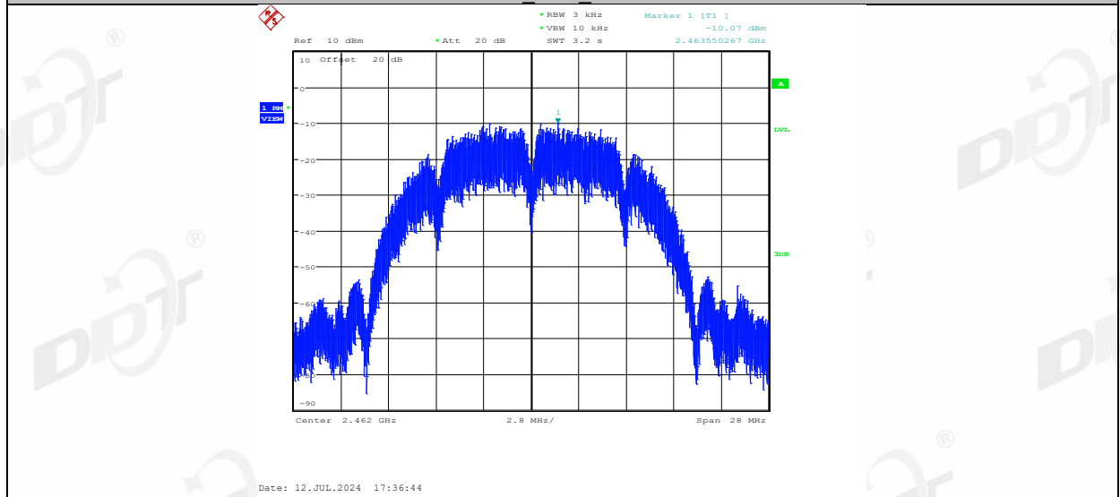
11B_Ant2_2462
