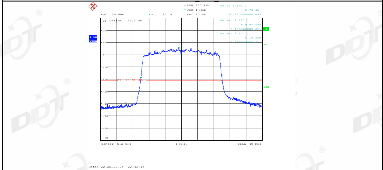
11AX20MIMO_Ant2_5200
