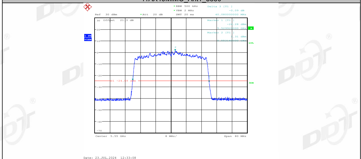
11AX40MIMO_Ant2_5550
