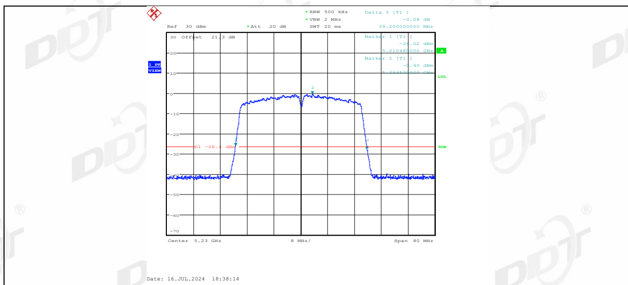
11N40MIMO Ant2 5230
