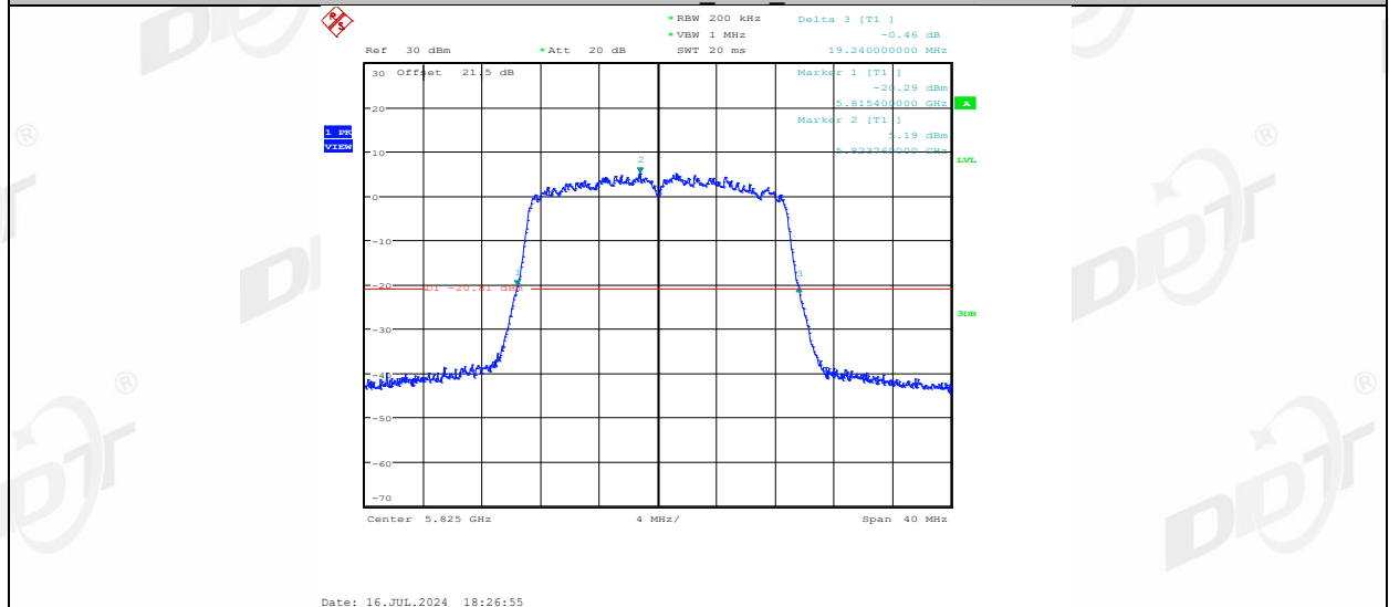
11N20MIMO_Ant2_5825
