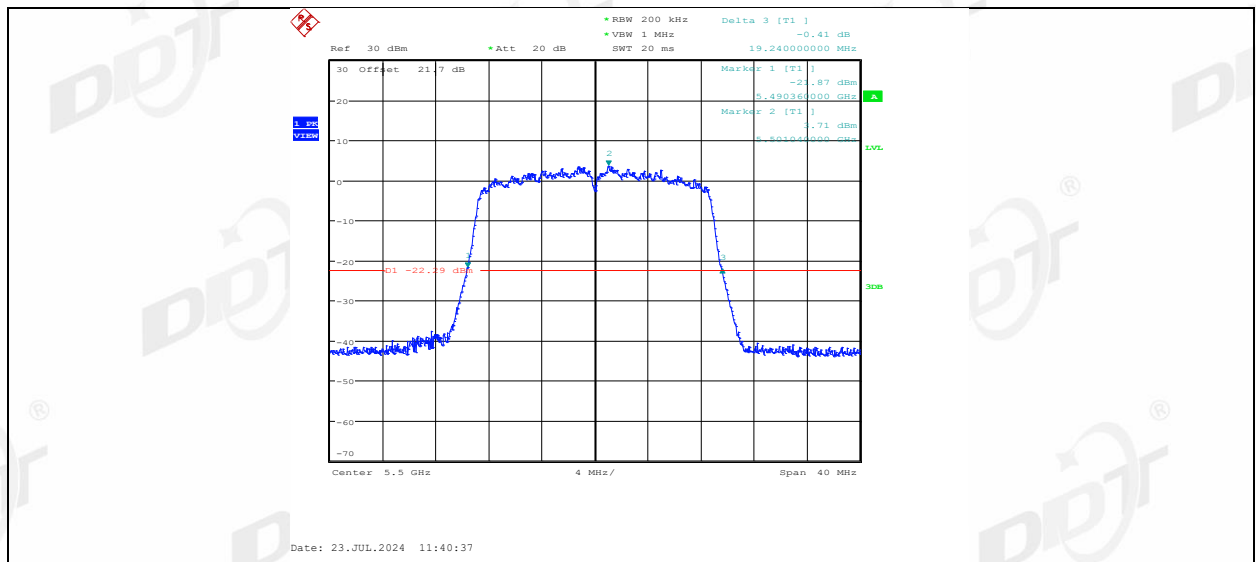
11AX20MIMO_Ant1_5580
