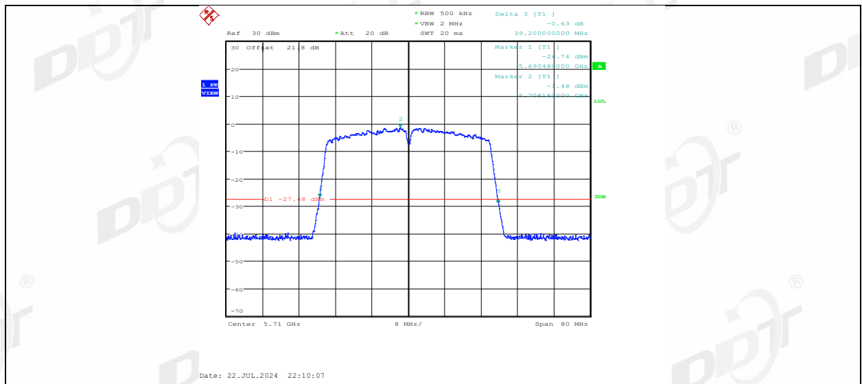
11N40MIMO_Ant2_5710
