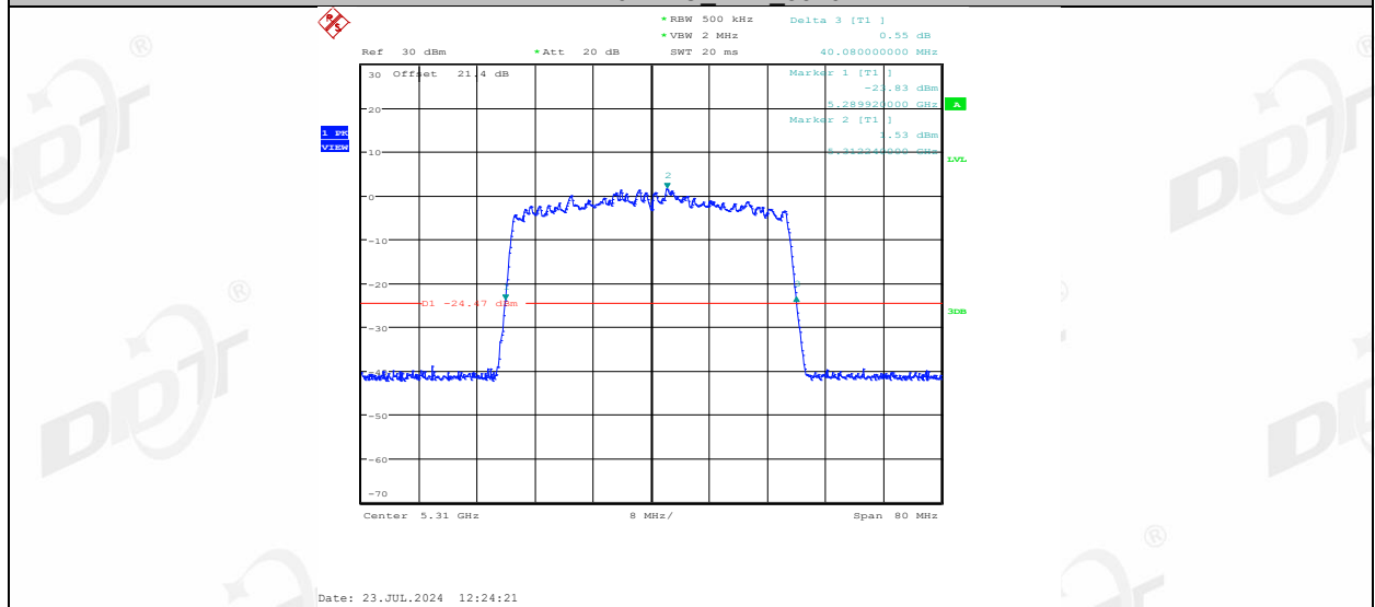
11AX40MIMO_Ant2_5310
