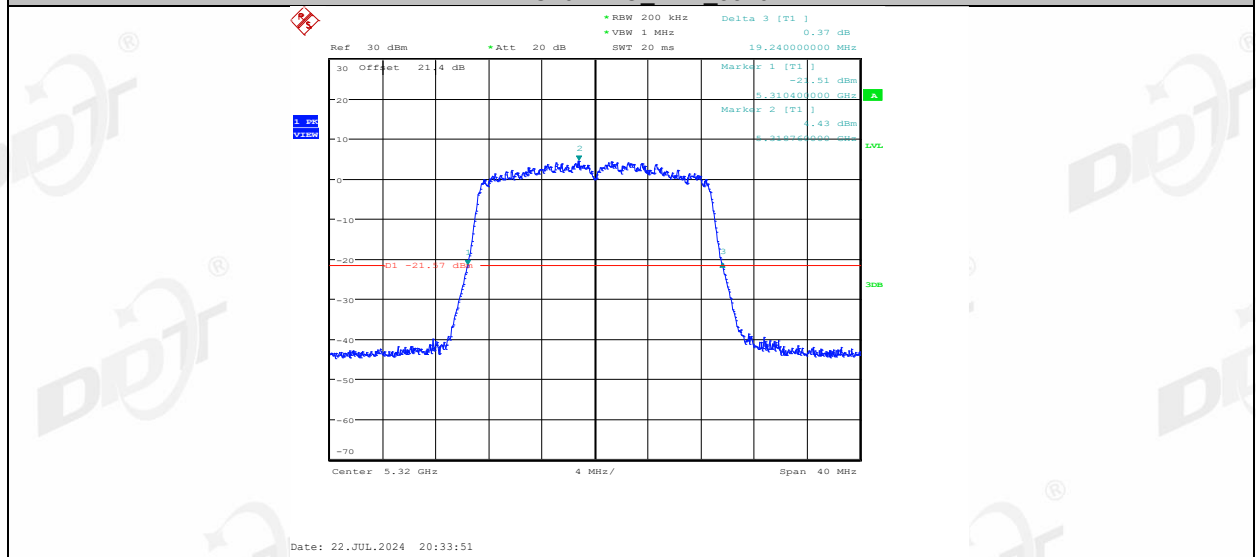
11AC20MIMO_Ant2_5320
