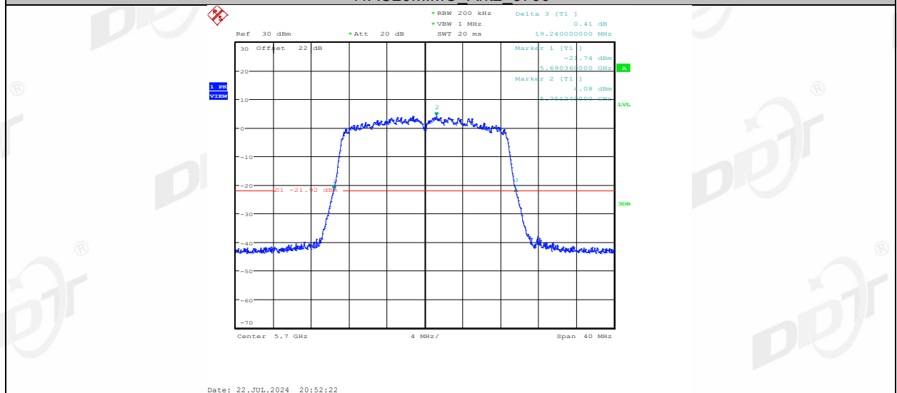
11AC20MIMO_Ant1_5720
