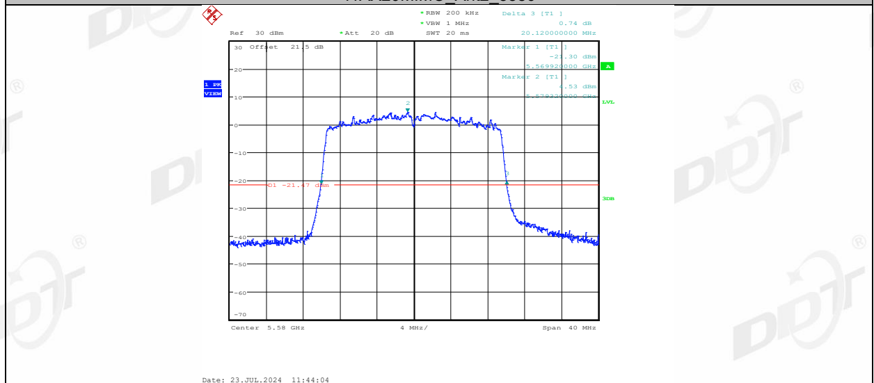
11AX20MIMO Ant1 5700
