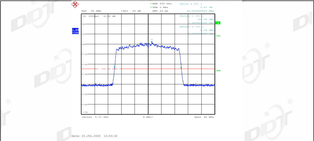
11AX40MIMO_Ant2_5710
