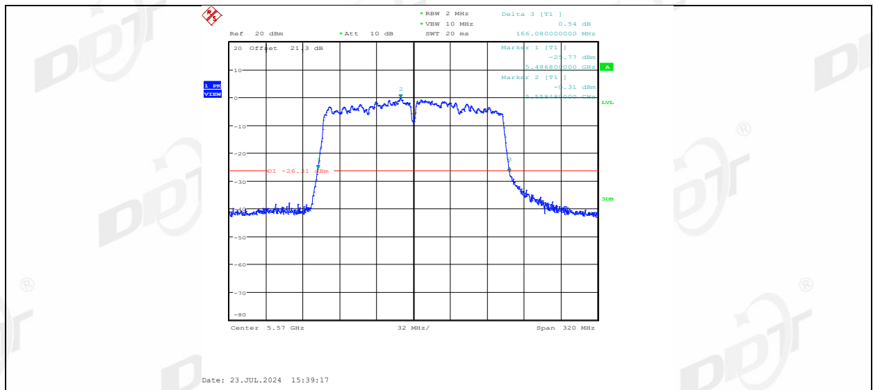
11AC160MIMO_Ant2_5570
