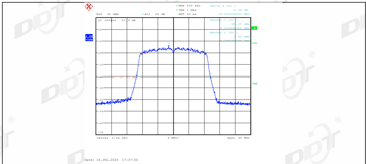
11N20MIMO_Ant2_5240
