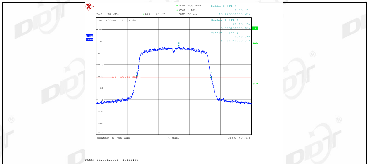
11N20MIMO_Ant2_5785
