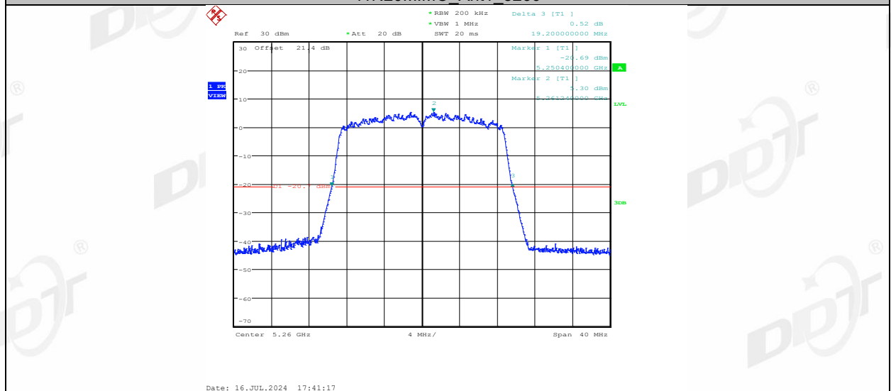
11N20MIMO_Ant2_5260
