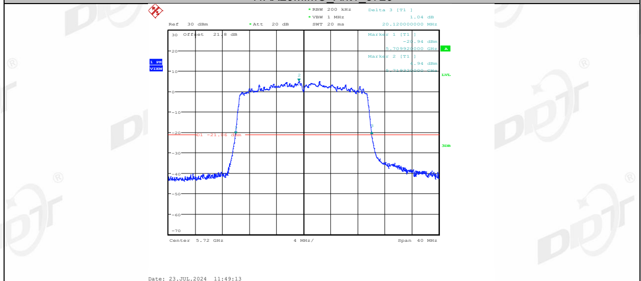
11AX20MIMO Ant2 5720
