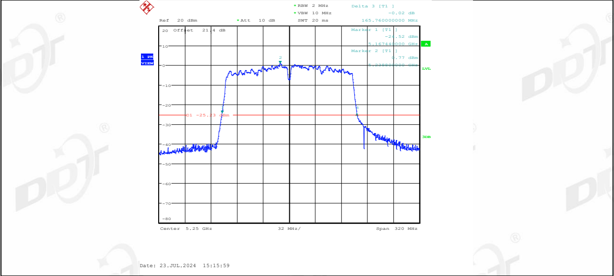
11AC160MIMO_Ant2_5250
