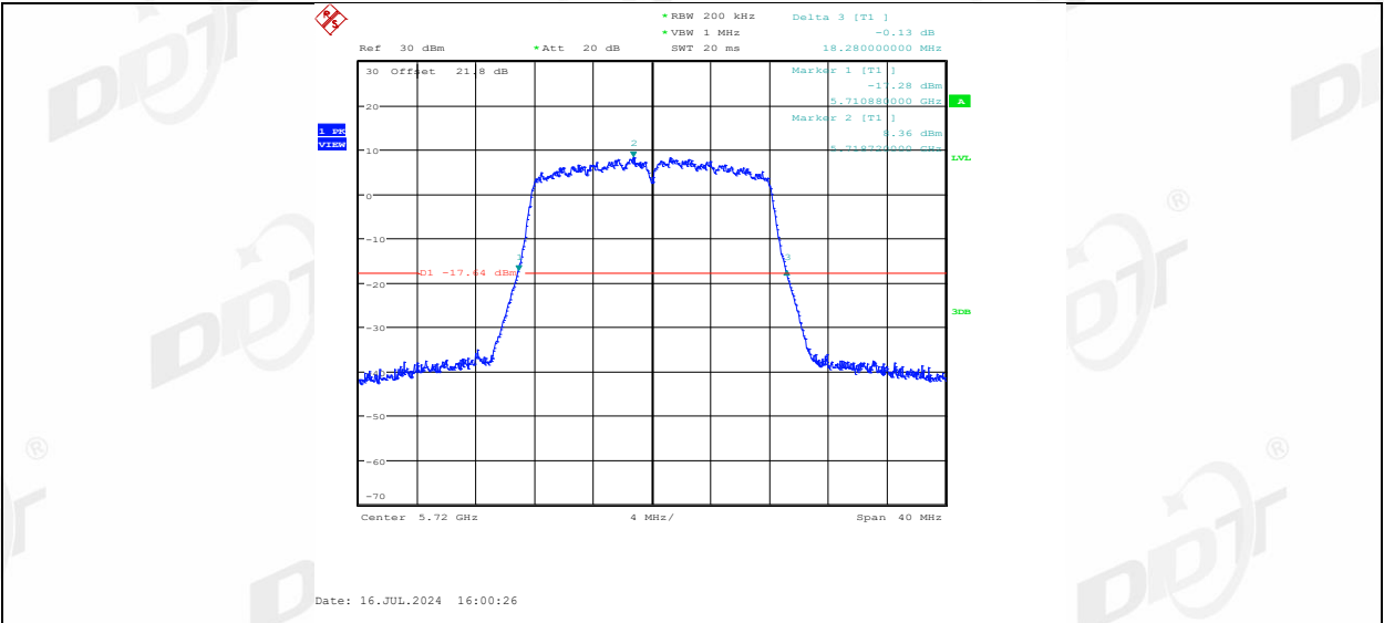
11A_Ant2_5720
