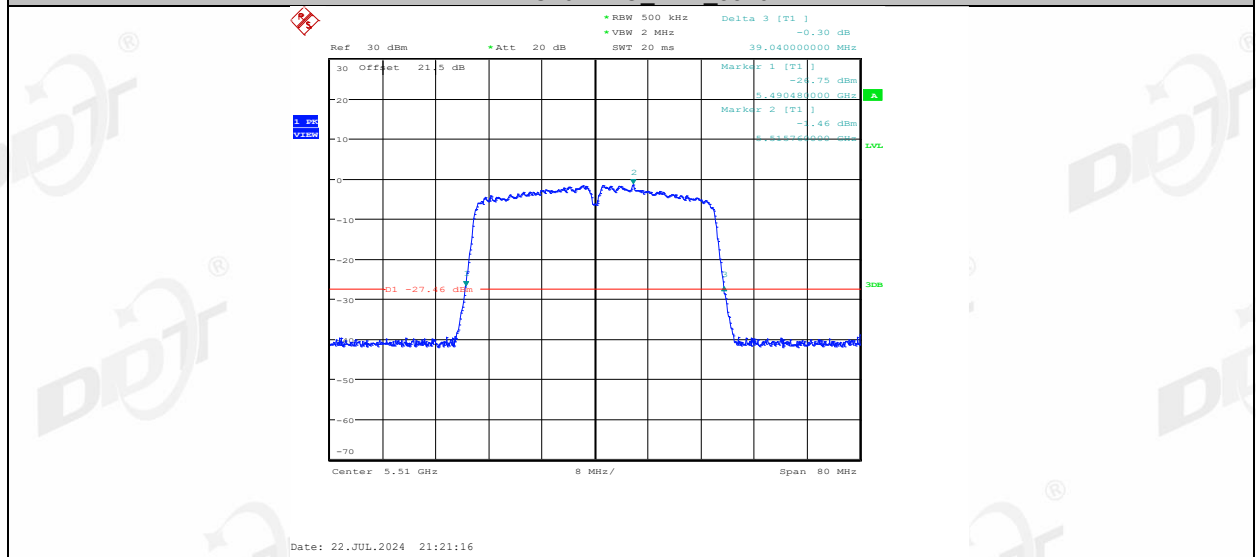
11AC40MIMO_Ant2_5510
