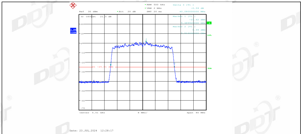
11AX40MIMO_Ant2_5510
