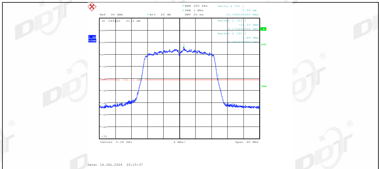
11AC20MIMO_Ant2_5180
