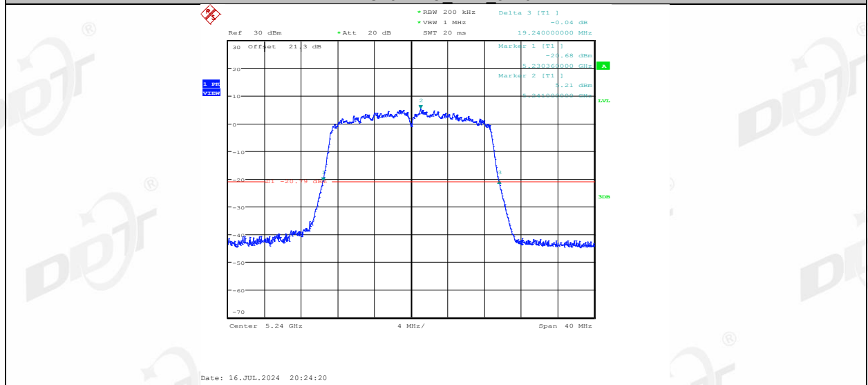
11AC20MIMO_Ant2_5240
