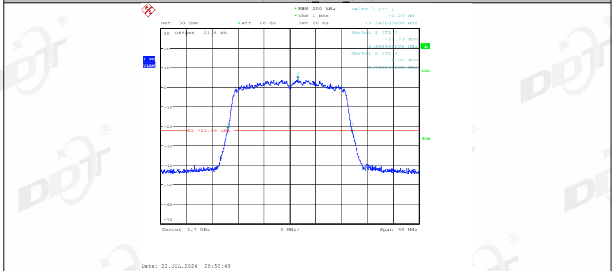
11AC20MIMO_Ant2_5700
