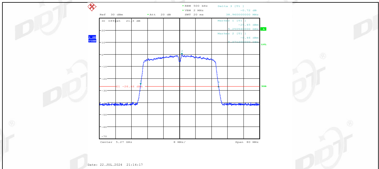
11AC40MIMO_Ant2_5270
