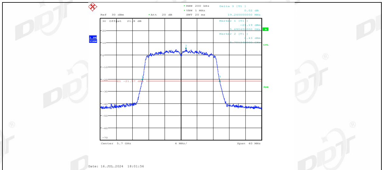
11N20MIMO_Ant2_5700
