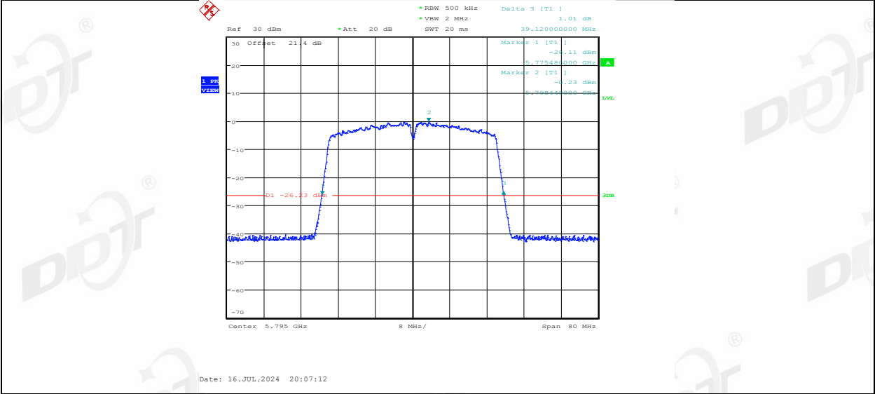
11N40MIMO_Ant2_5795
