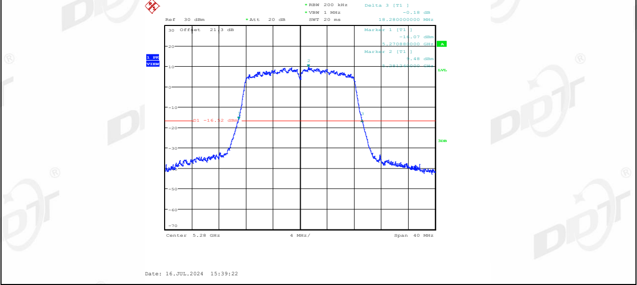
11A_Ant2_5280
