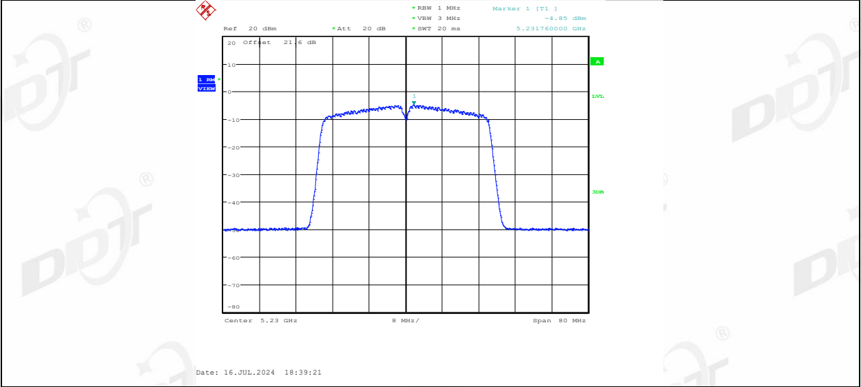
11N40MIMO_Ant2_5230
