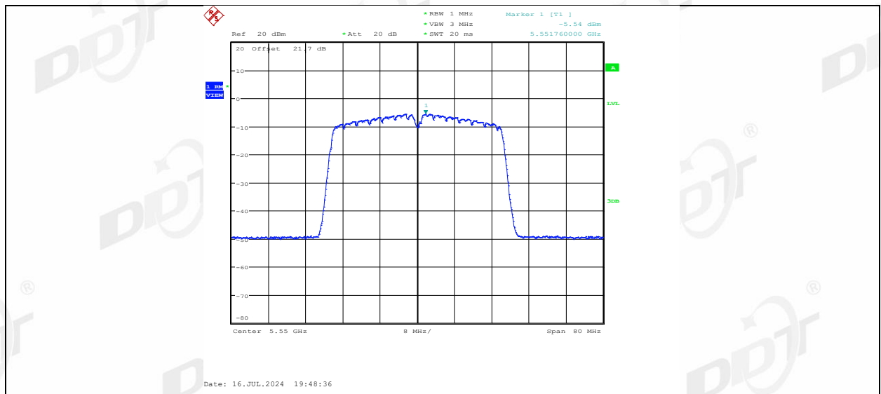
11N40MIMO_Ant2_5550
