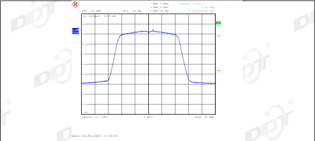
11N20MIMO_Ant2_5200
