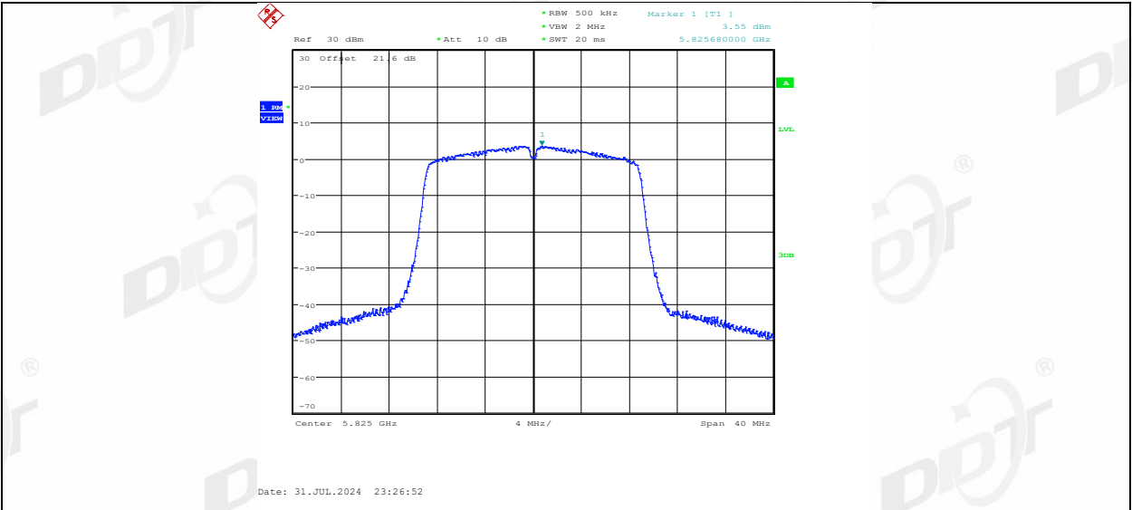
11N20MIMO_Ant2_5825
