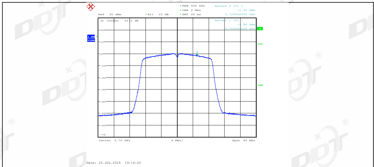
11AC20MIMO_Ant1_5745
