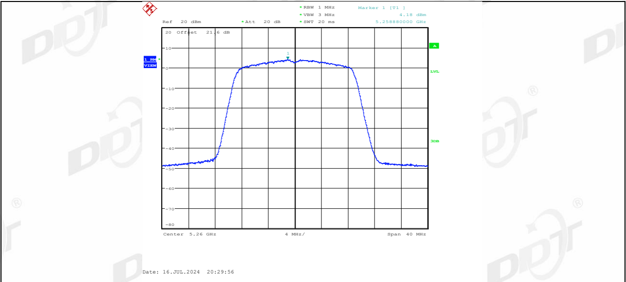
11AC20MIMO_Ant2_5260
