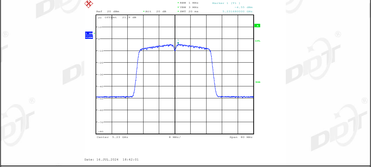
11N40MIMO_Ant1_5270
