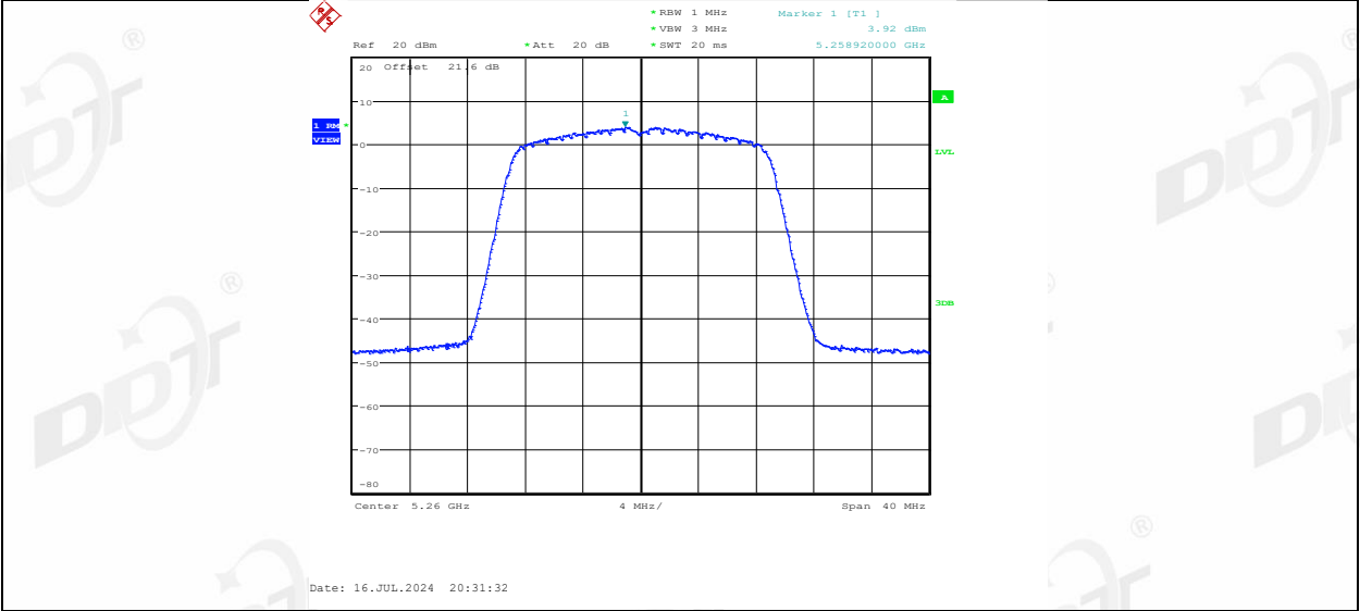
11AC20MIMO_Ant1_5280
