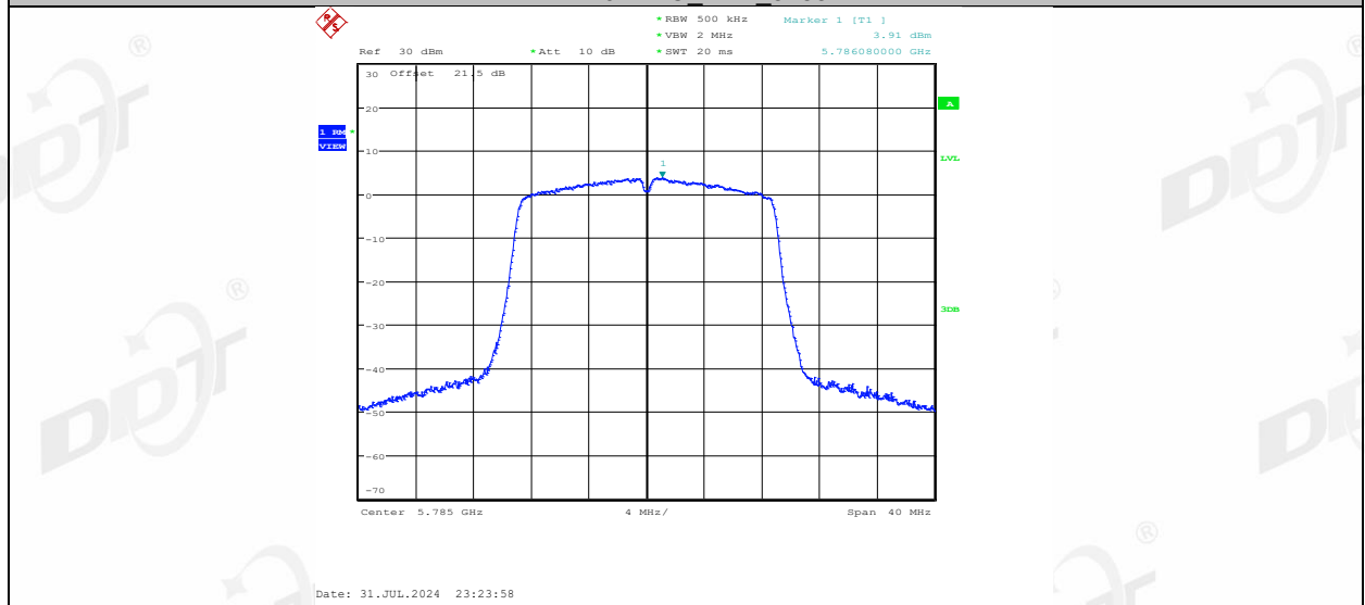
11N20MIMO_Ant2_5785
