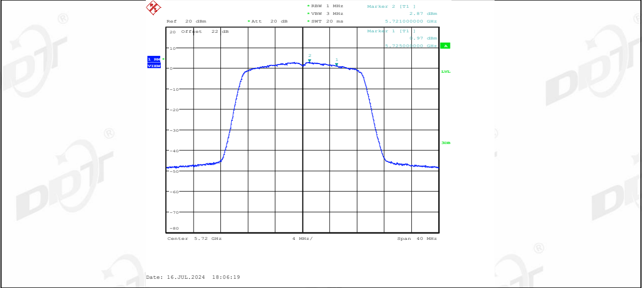
11N20MIMO_Ant2_5720_UNII-2C
