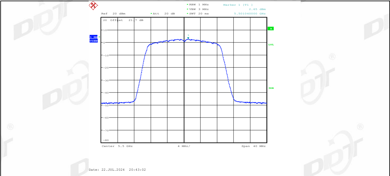
11AC20MIMO_Ant2_5500
