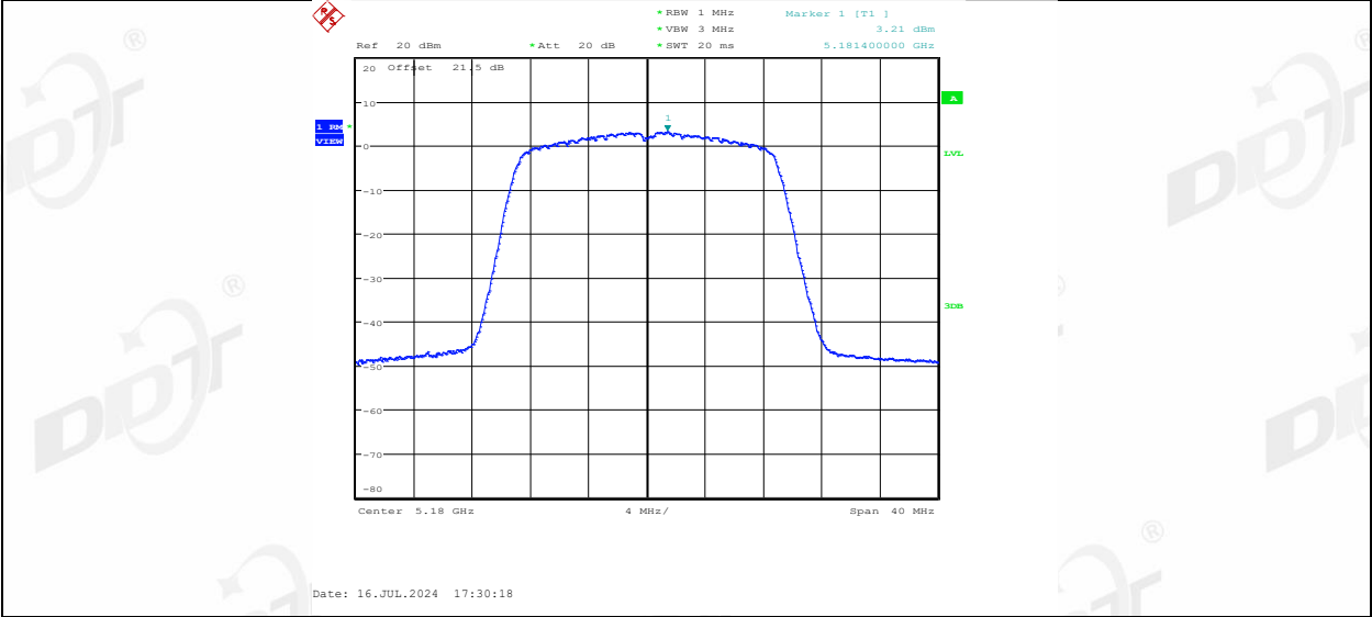
11N20MIMO_Ant2_5180
