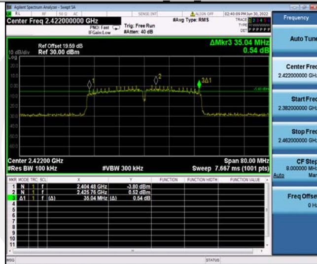
11N40SISO_Ant2_2422
