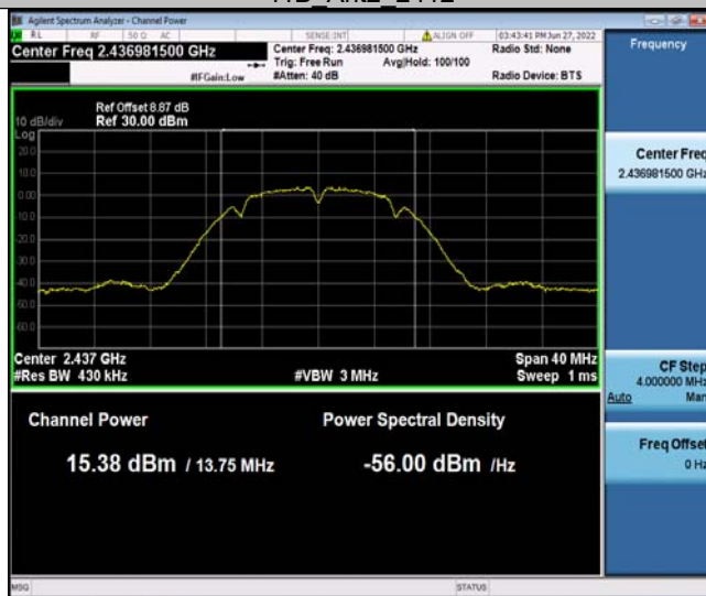
11B_Ant1_2437
