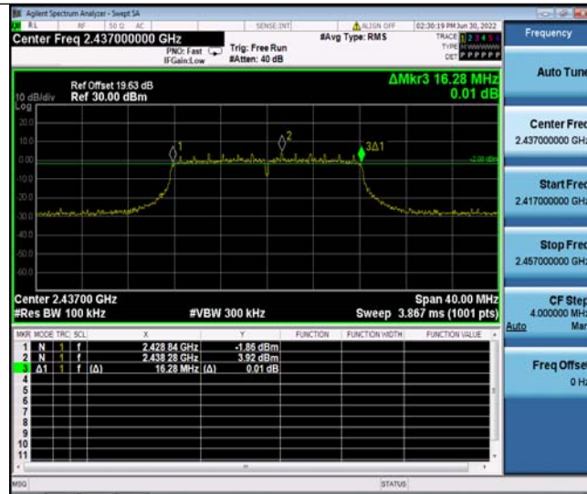
11G_Ant2_2437
