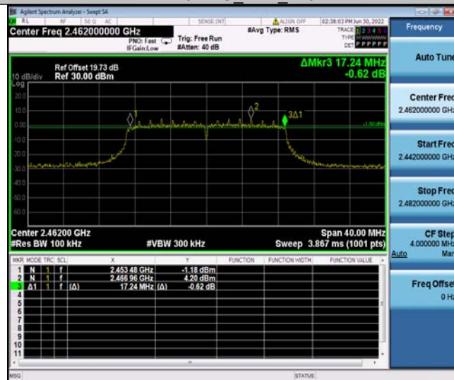
11N20SISO_Ant2_2462
