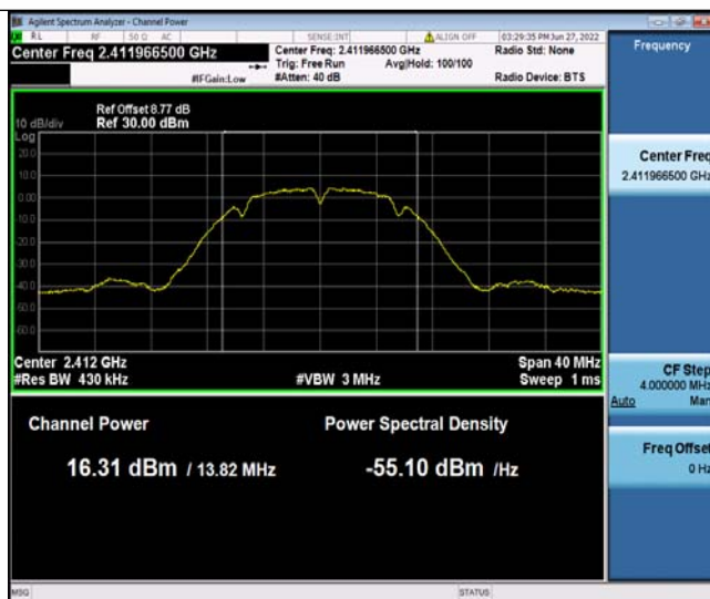
11B_Ant1_2412
