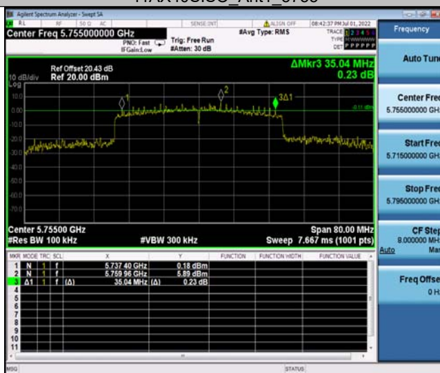
11AX40SISO_Ant2_5755
