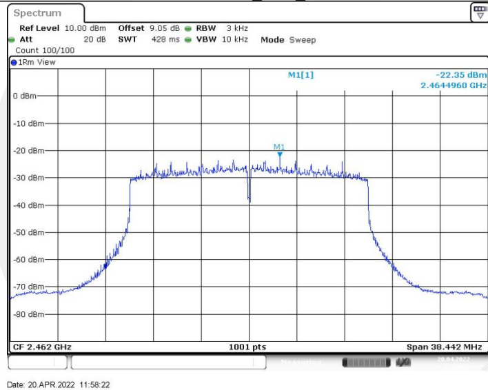
11AX20SISO_Ant2_2462
