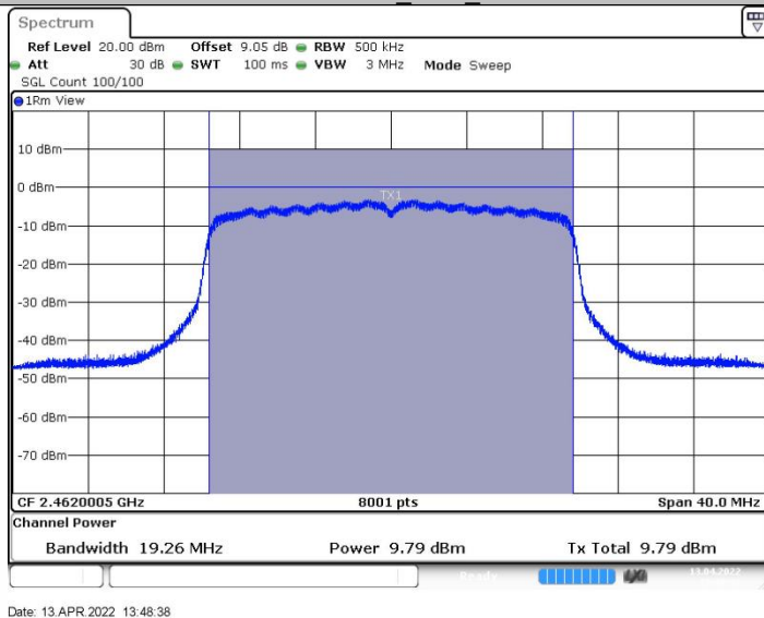
11AX20SISO_Ant2_2462
