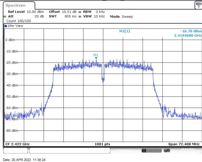
11N40SISO_Ant2_2422
