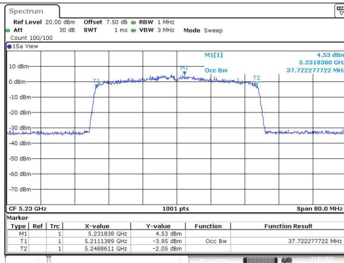
11AX40SISO_Ant2_5230
