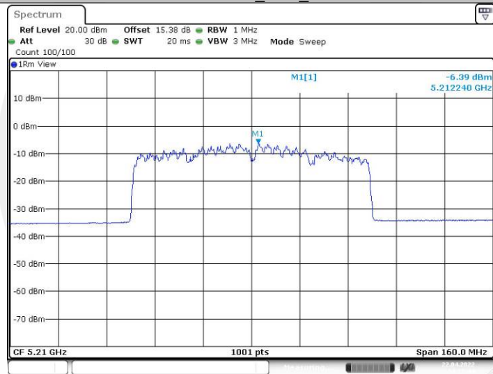
11AX80SISO_Ant2_5210
