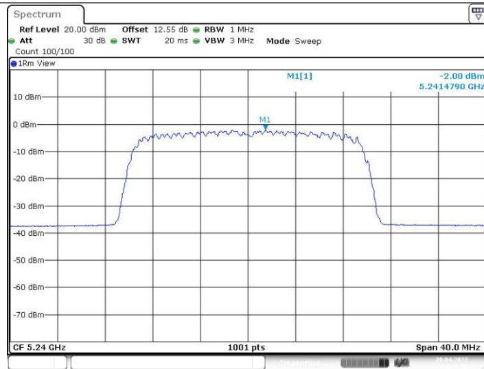
11AX20SISO_Ant2_5240
