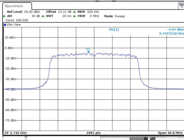
11AX20SISO_Ant2_5745
