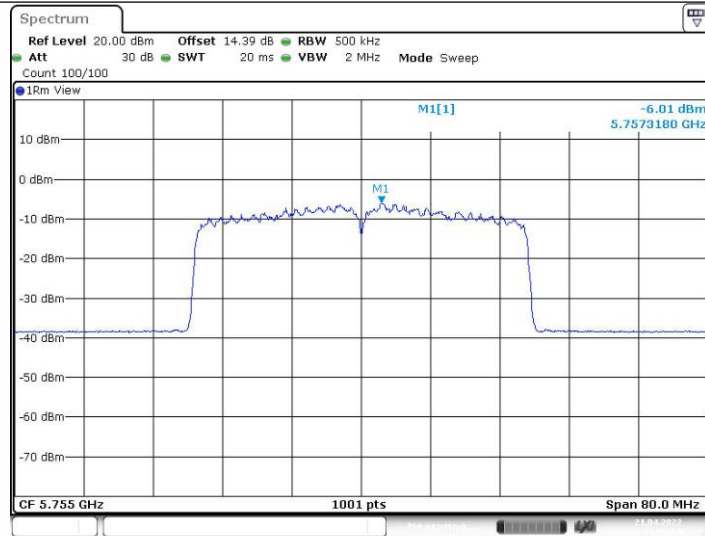
11AX40SISO_Ant2_5755
