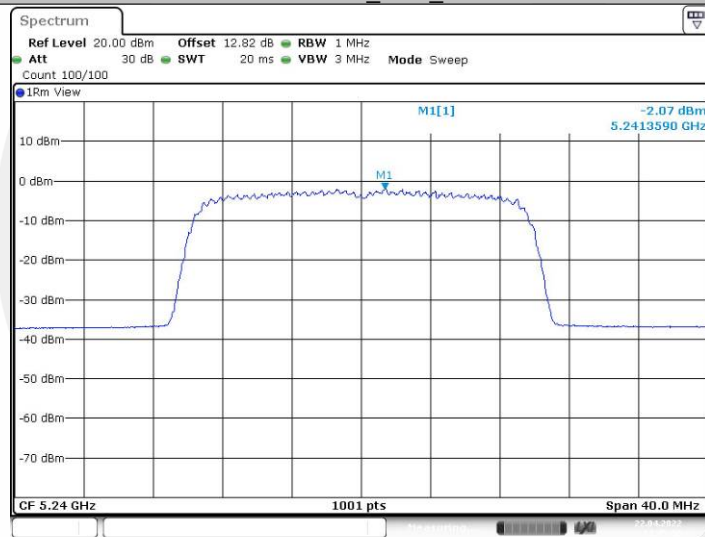
11AX20SISO_Ant2_5240
