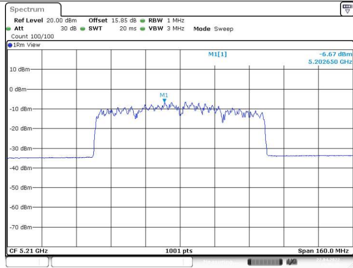
11AX80SISO_Ant2_5210
