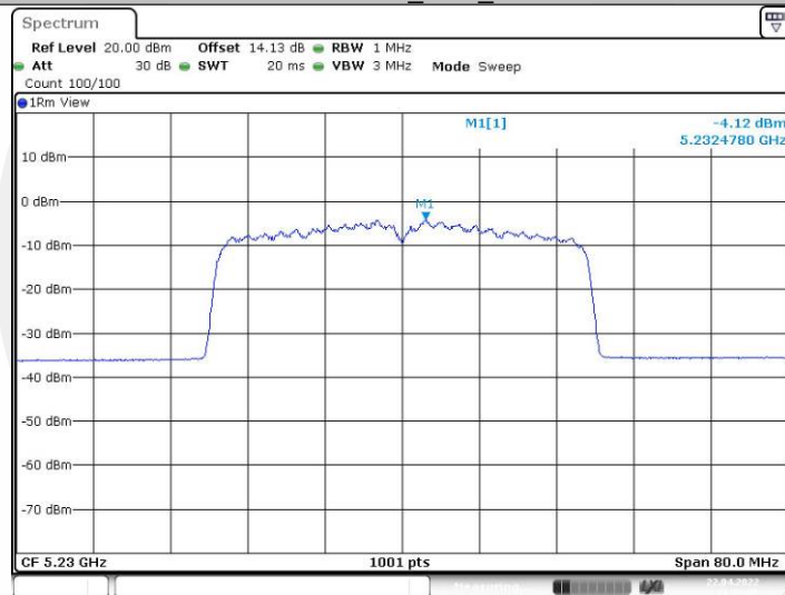
11AX40SISO_Ant2_5230
