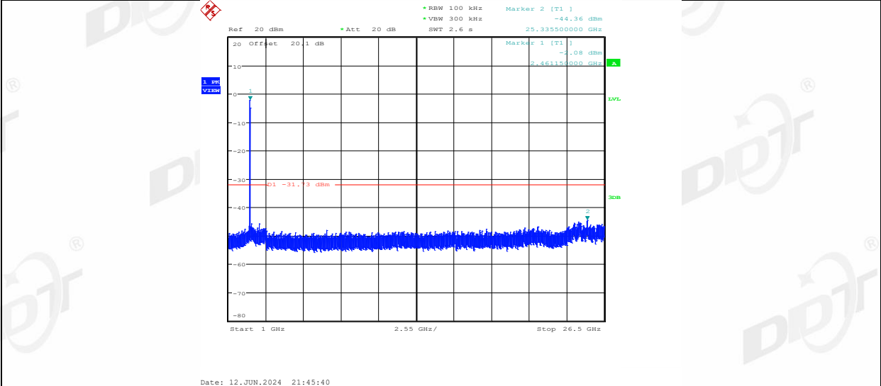
11N40MIMO_Ant1_2422_0~Reference
