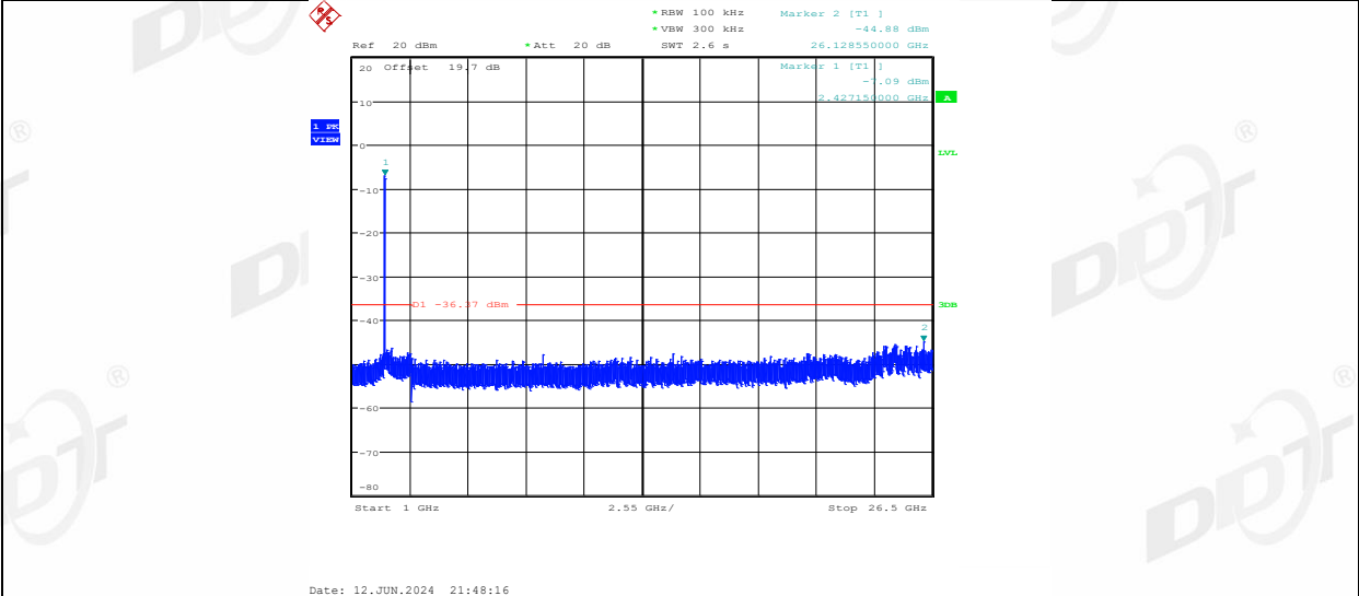
11N40MIMO_Ant2_2422_0~Reference
